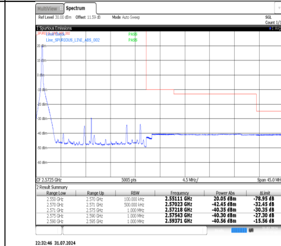
Band7-20MHz-QPSK-21350-1RB#99-PASS
