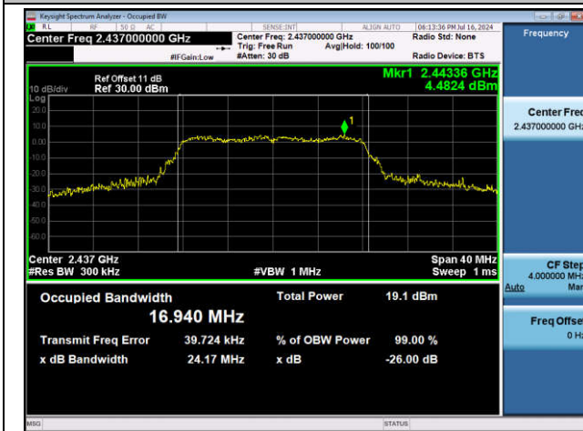
11G-Ant1-2437
