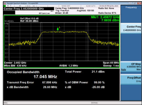
11G-Ant1-2462
