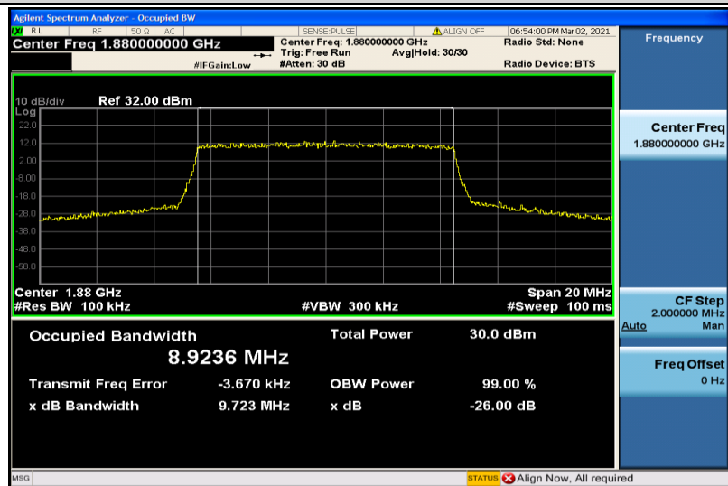
Band2-10MHz-QPSK-18900-50RB#0-8.9236
