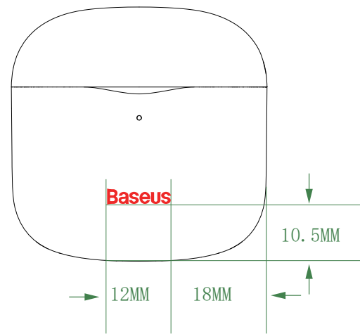
前视图
