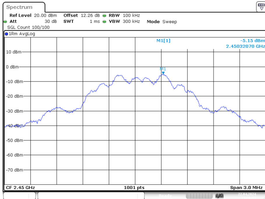
PSD NVNT BLE 1M 2450MHz Ant1
