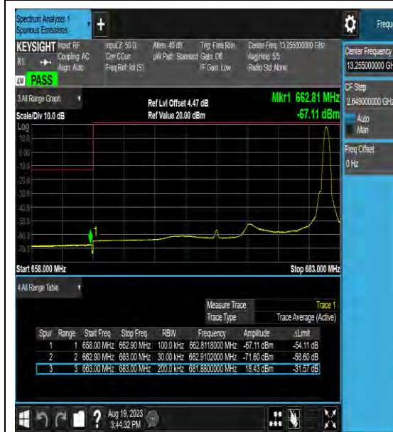
Band71_20MHz_QPSK_133222_100RB#0
