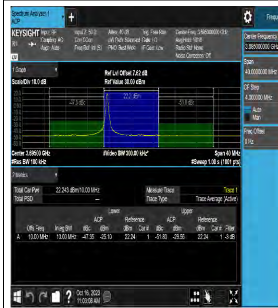
Band48-10MHz-QPSK-56690-1RB#49-PASS
