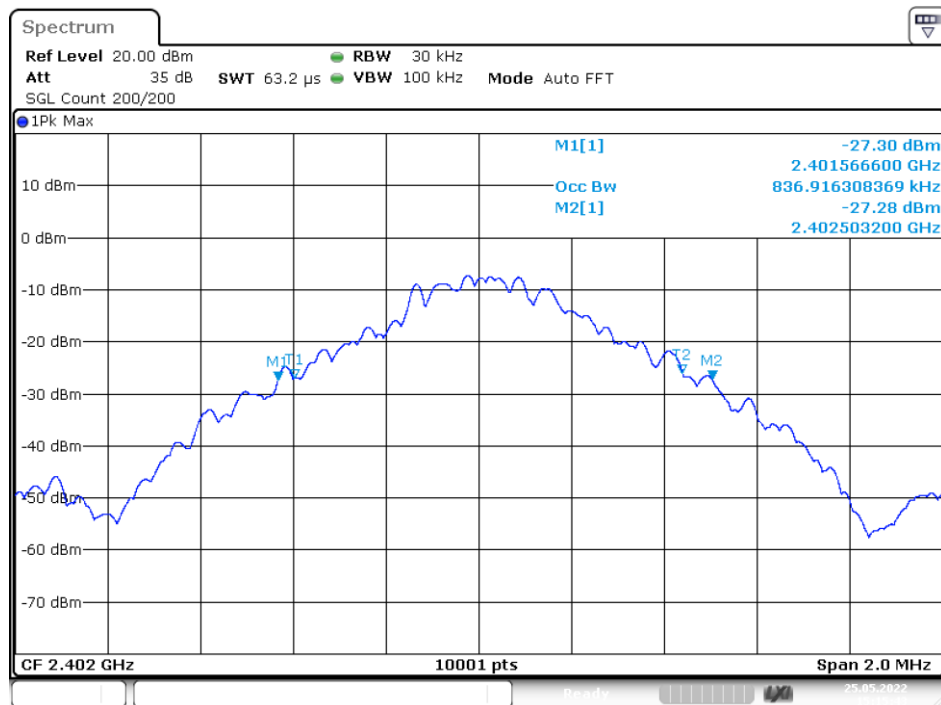
20dB NVNT 1-DH5 2402MHz Ant1
