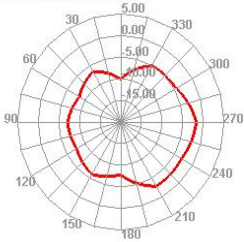
2400.000MHz E1
