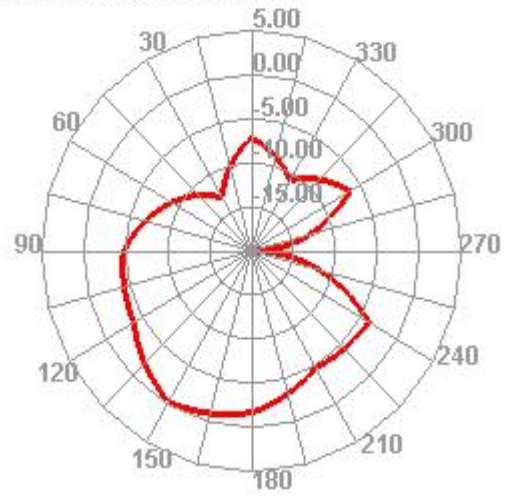
2400.000MHz H
