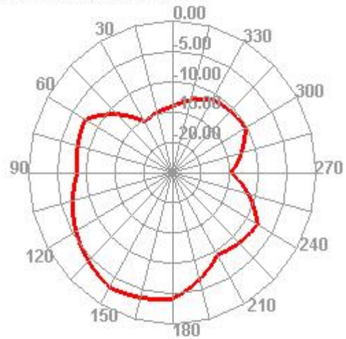
2500.000MHz H
