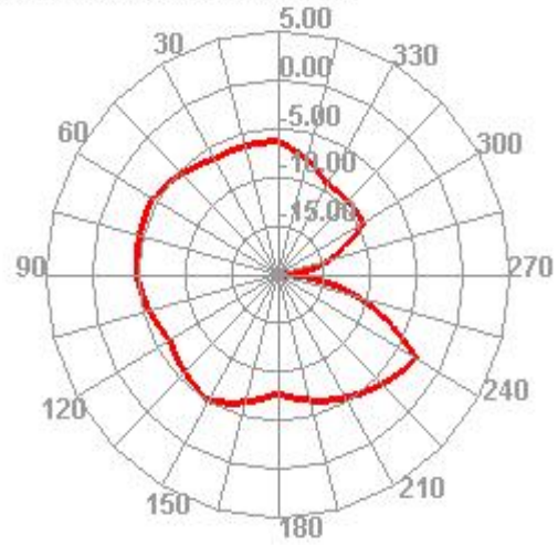
2400.000MHz E2
