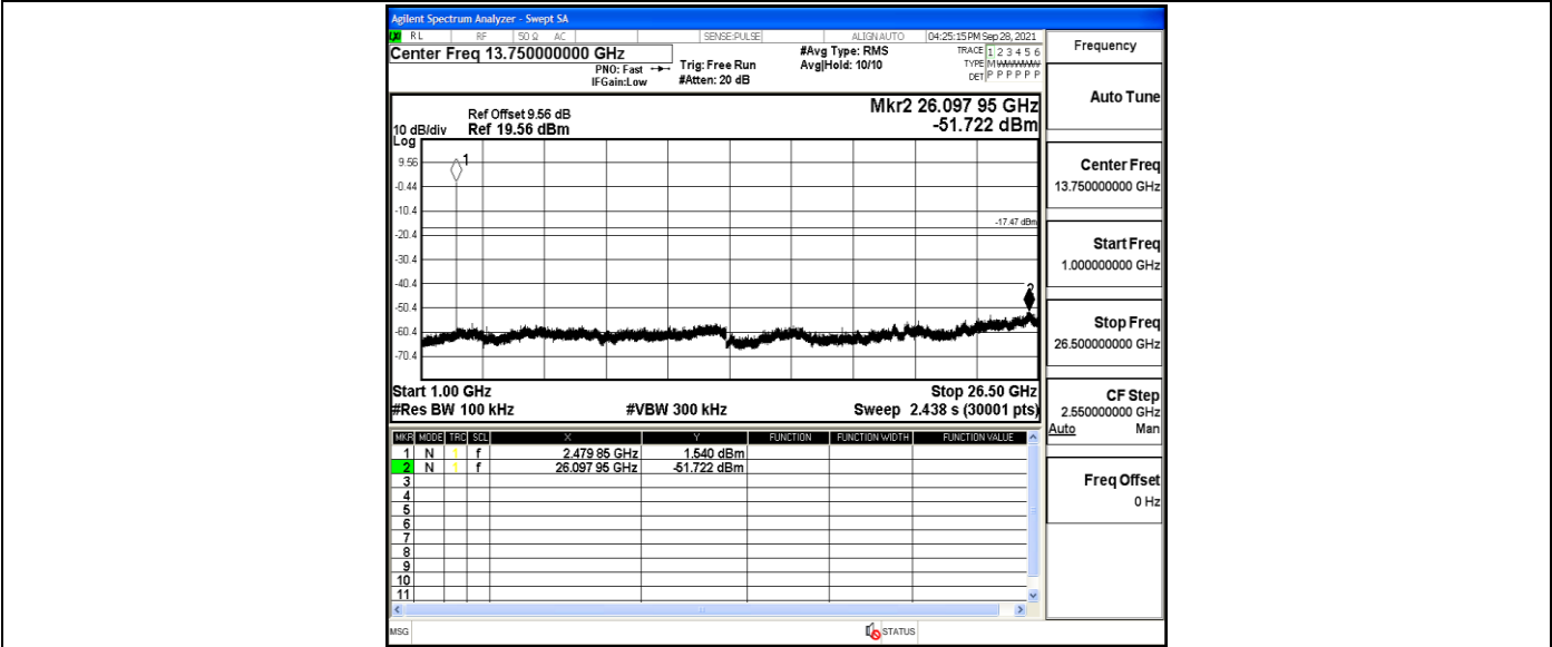
BLE_1M_Ant1_2480_1000~26500
