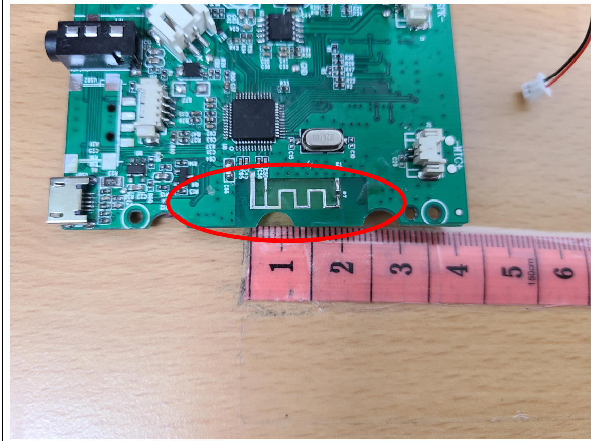
Antenna
