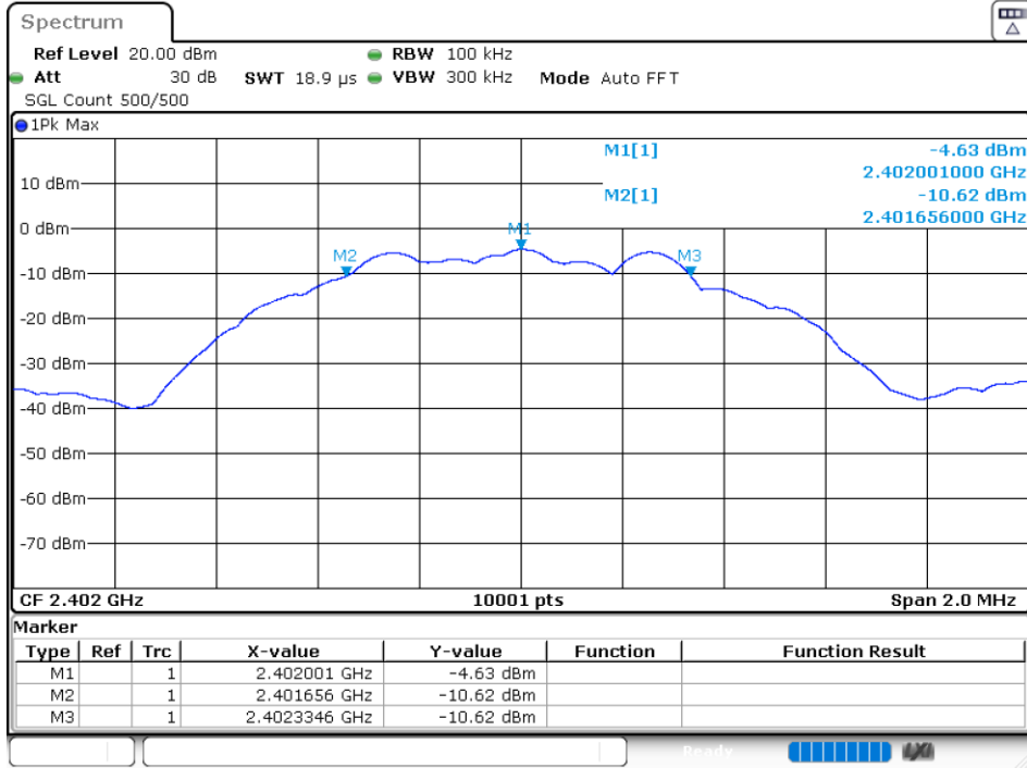
-6 dB BW NVNT BLE 2402MHz Ant2
