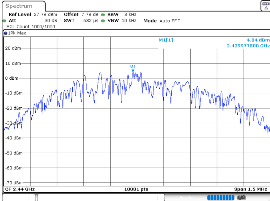
PSD NVNT BLE 2440MHz Ant2
