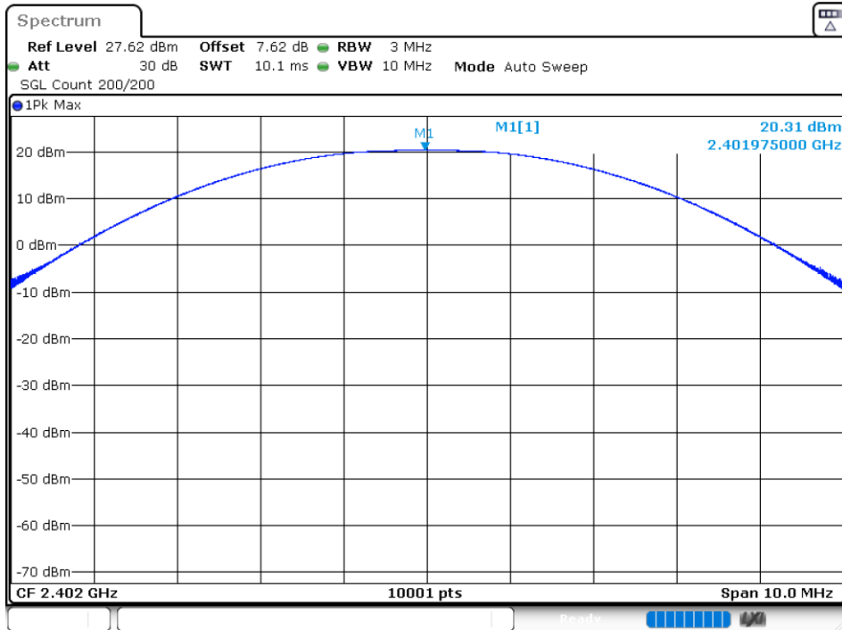
Power NVNT BLE 2402MHz Ant2
