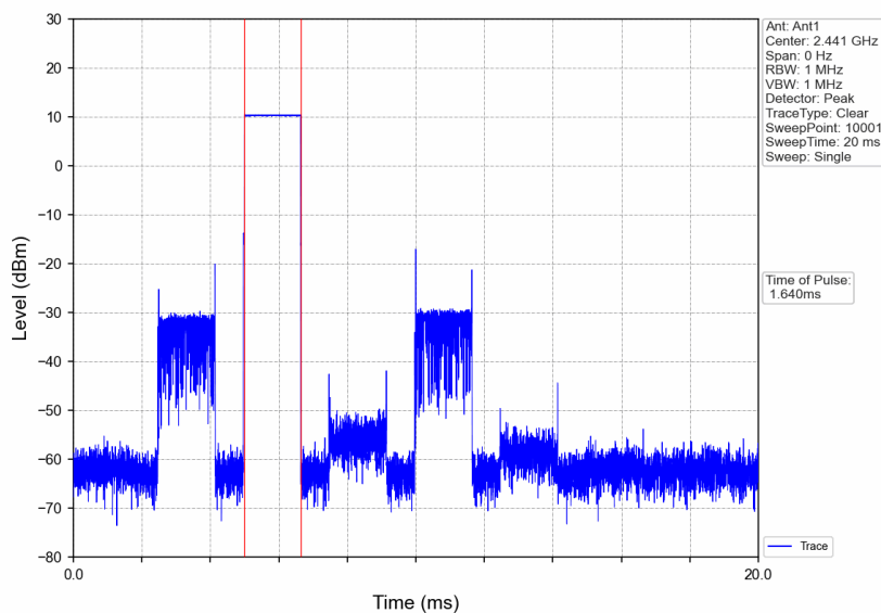
GFSK_DH3_HOPP_Ant1_NTNV
