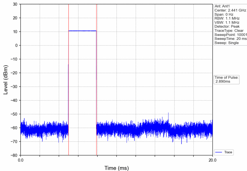
GFSK_DH5_HOPP_Ant1_NTNV
