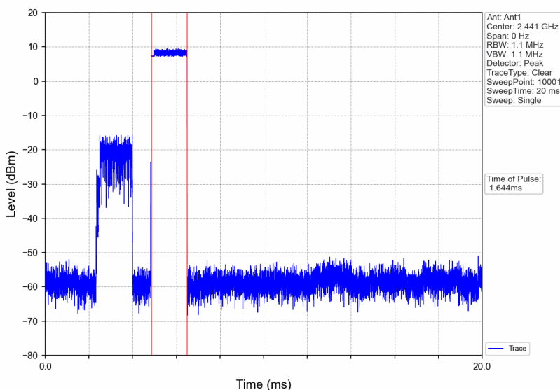
8DPSK_3DH3_HOPP_Ant1_NTNV
