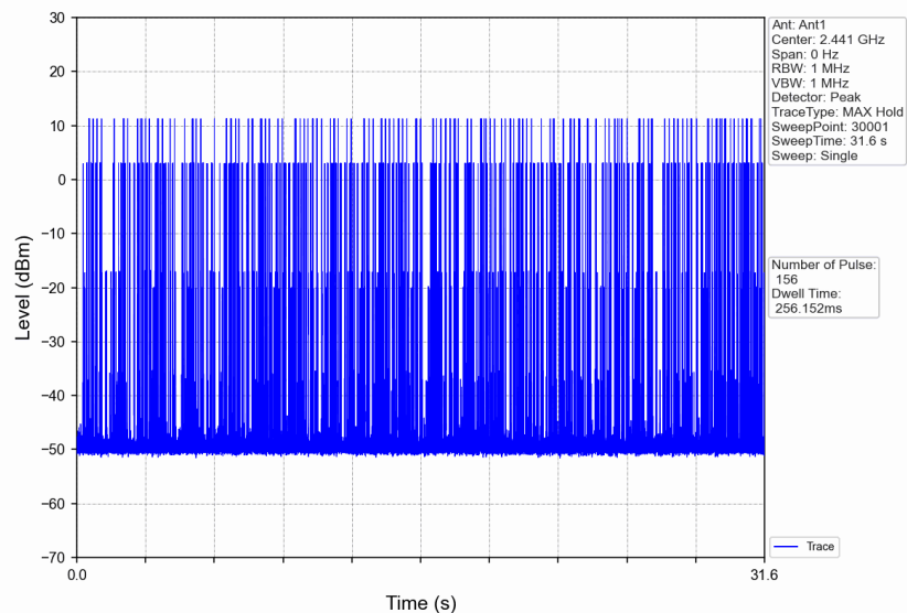
GFSK_DH3_HOPP_Ant1_NTNV
