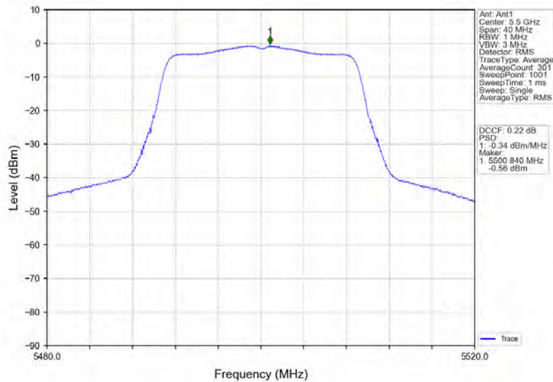
802.11ac(VHT20)_LCH_5500MHz_Ant1_NTNV
