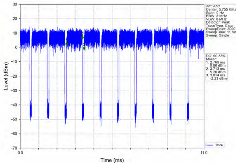
802.11n(HT40)_LCH_5755MHz_Ant1_NTNV
