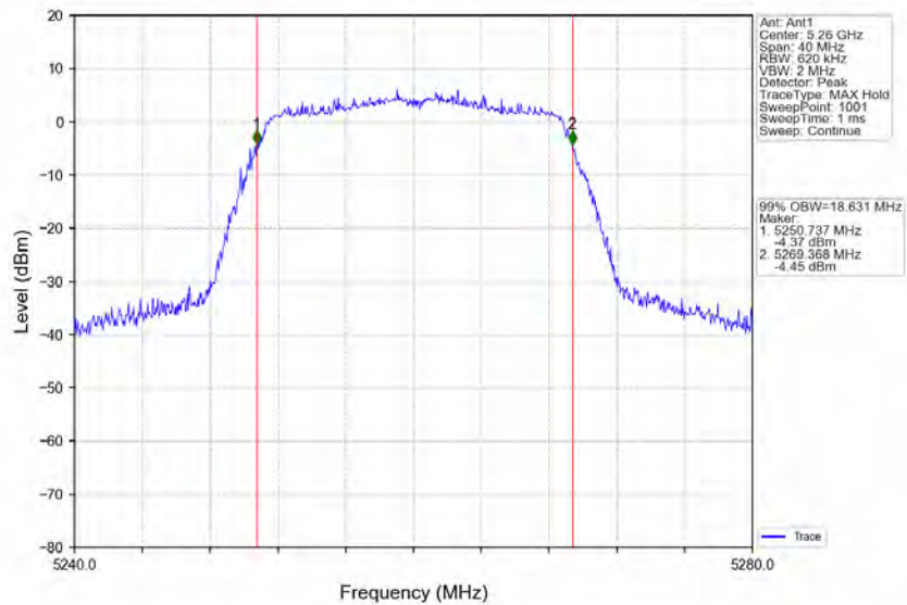
802.11n(HT20)_LCH_5260MHz_Ant1_NTNV
