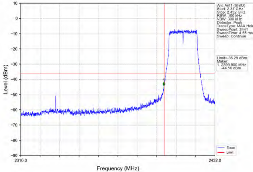
802.11n(HT20)_LCH_2412MHz_Ant1 (SISO)_NTNV
