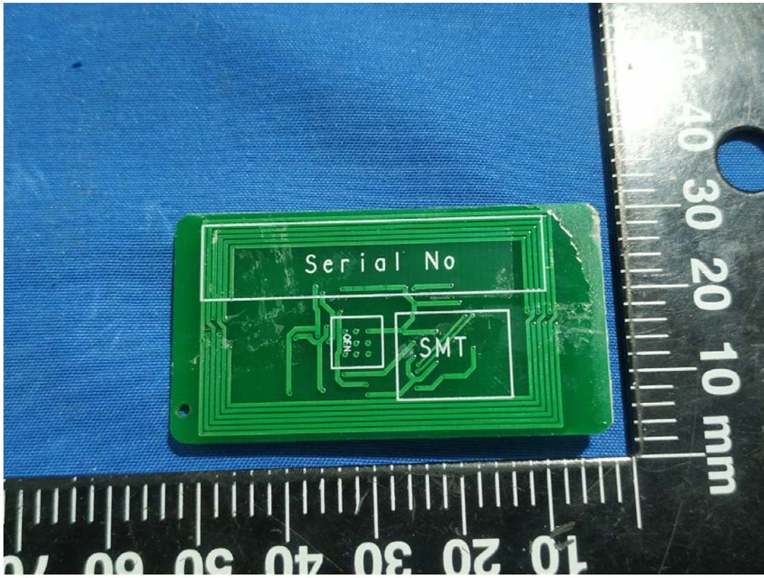
NFC Antenna
