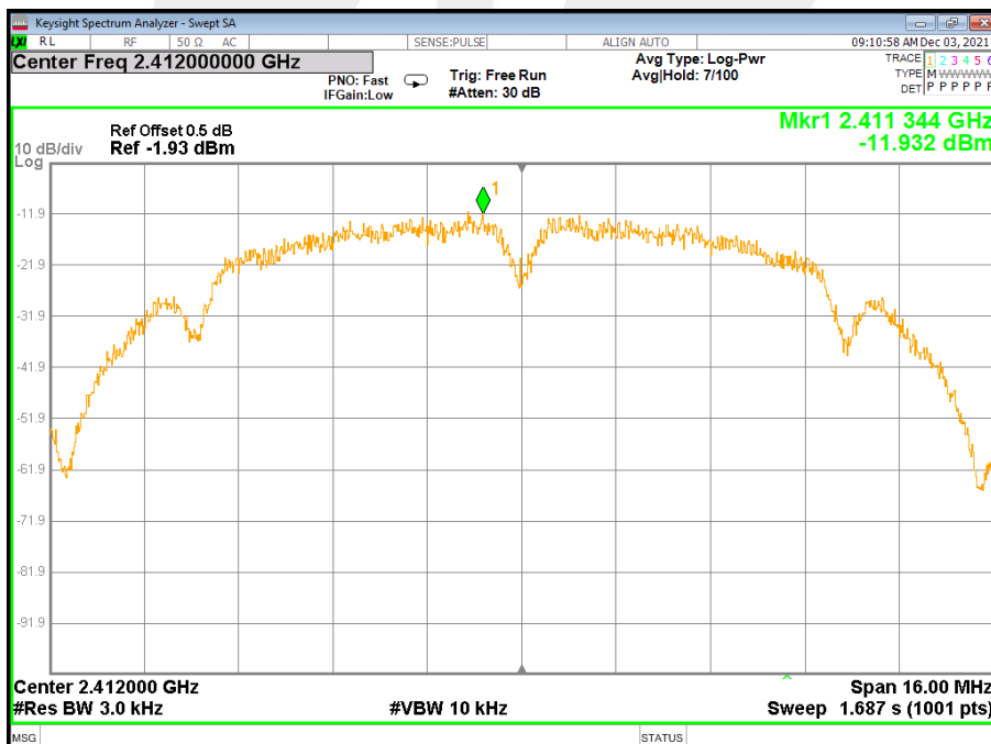
802.11 b TX CH01
