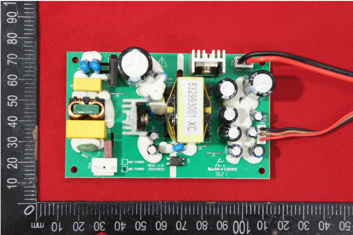
Mains PCB
