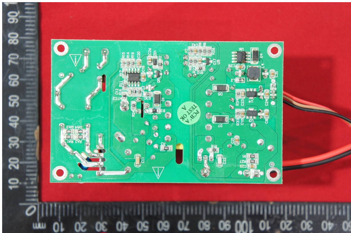
Mains PCB
