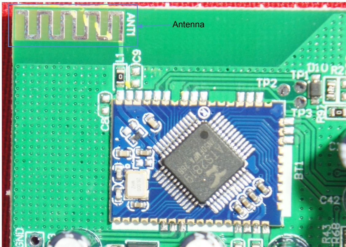
Bluetooth module
