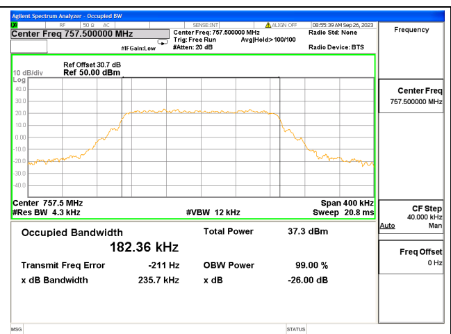
757MHz-758MHz / 15KHz / QPSK/ Mid CH
