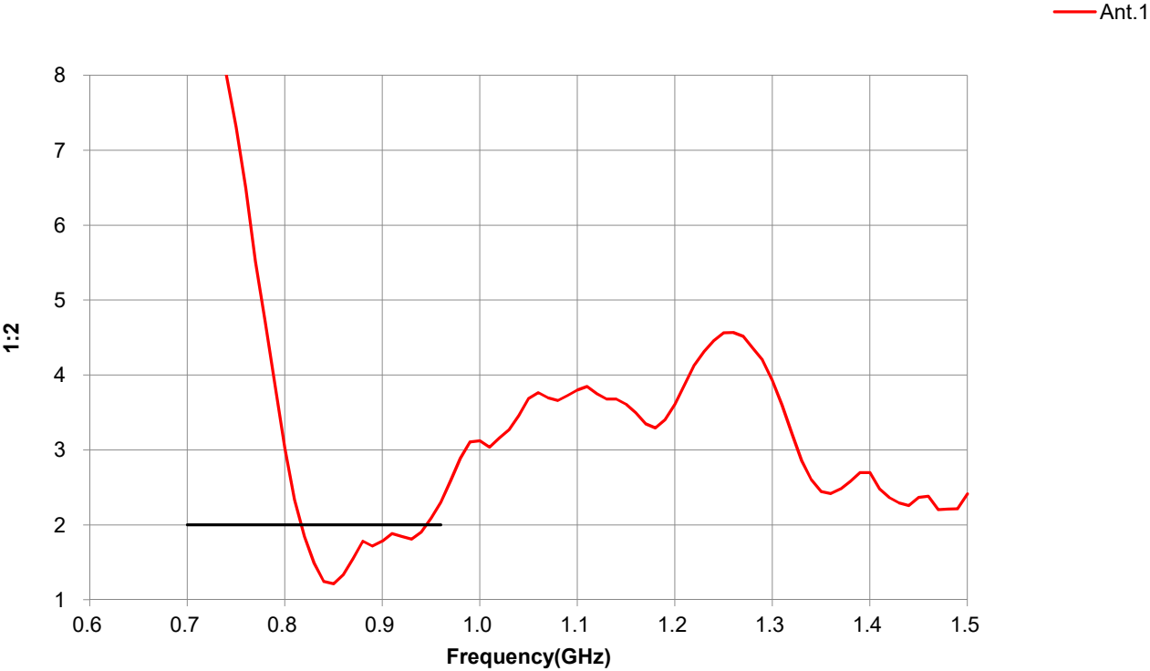
VSWR
