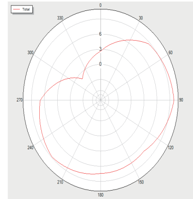
BLUETOOTH_Trp_V0 Total
