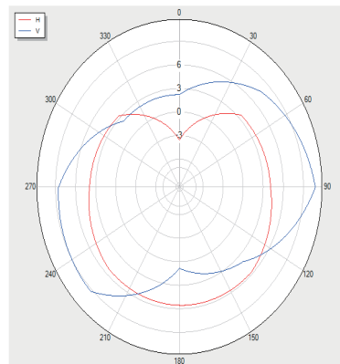
BLUETOOTH_Trp_V78 Polar
