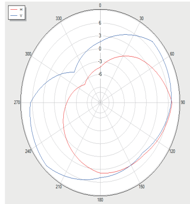
BLUETOOTH_Trp_V0 Polar
