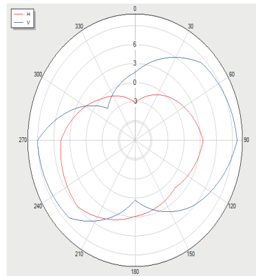
BLUETOOTH_Trp_V39 Polar
