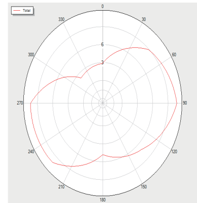
BLUETOOTH_Trp_V39 Total
