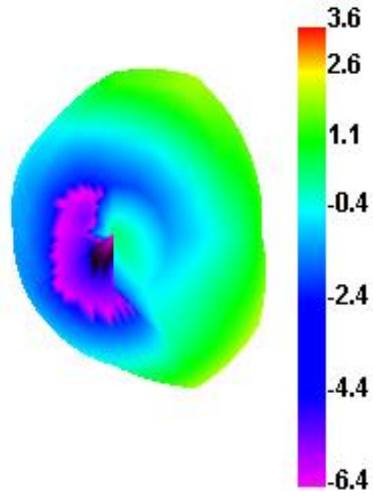
2450.000MHz E1
