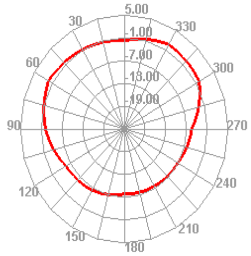
2450.000MHz H
