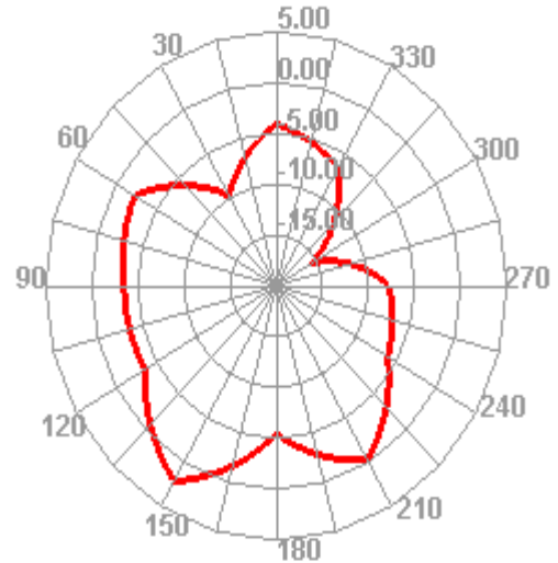
2500.000MHz E2
