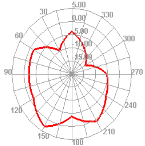
2450.000MHz E2
