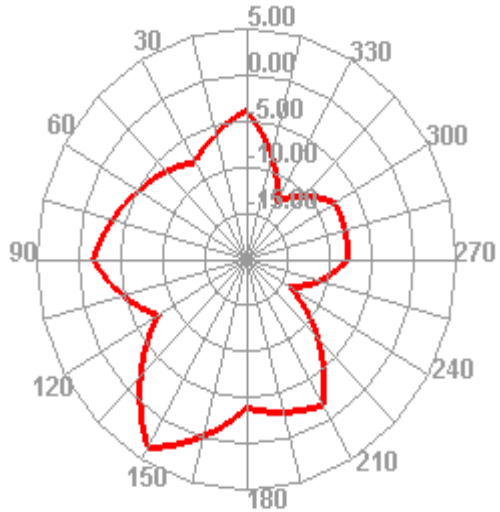
2450.000MHz E1
