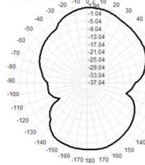
2400.0MHz Total(E1-XZ), Max= 2.26dBi
