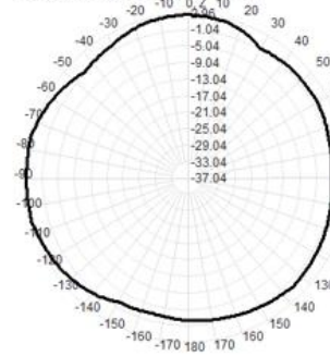
2400.0MHz Total(E2-YZ), Max= 2.96dBi
