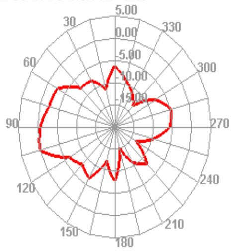
2450.000MHz E2
