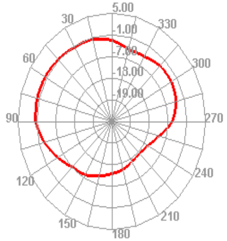
2450.000MHz H
