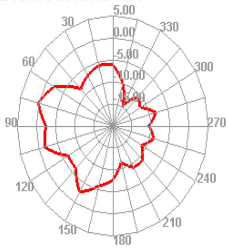
2450.000MHz E1
