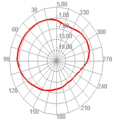
2500.000MHz H
