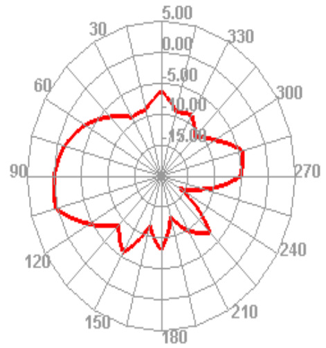
2500.000MHz E2
