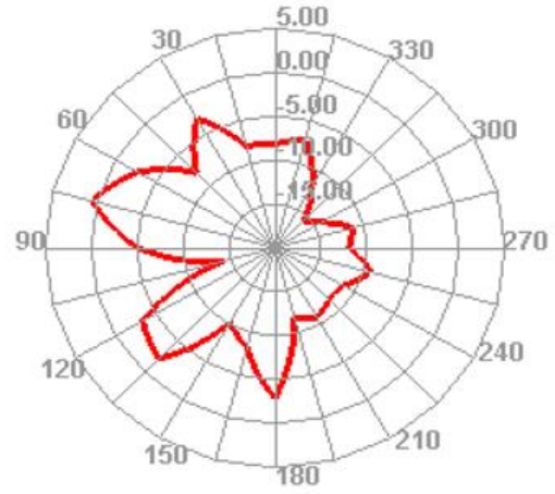
2500.000MHz E2
