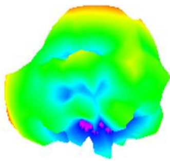
2450.000MHz
