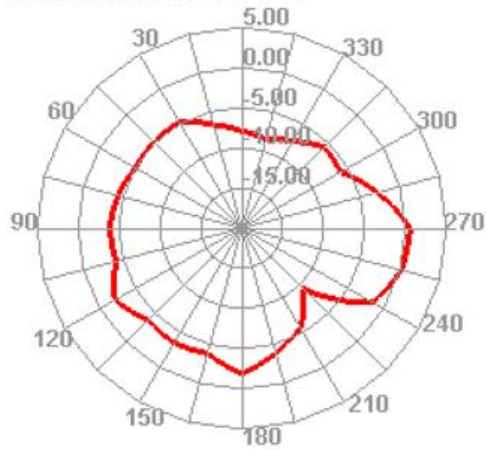
2400.000MHz E1
