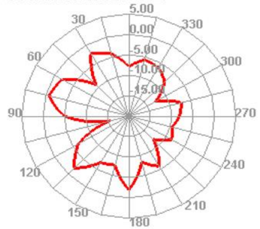
2400.000MHz E2
