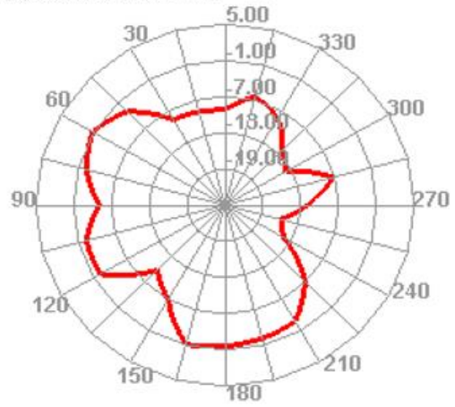
2500.000MHz E2
