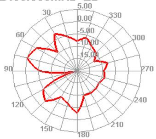
2450.000MHz E2
