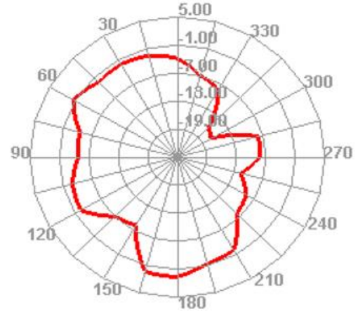
2400.000MHz H
