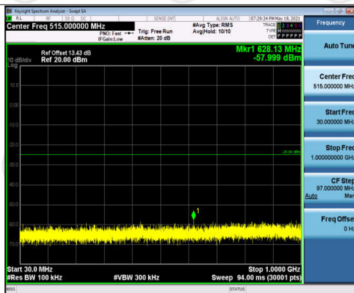
11G_Ant1_2472_30~1000
