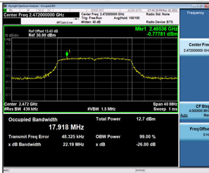
11N20SISO_Ant1_2472
