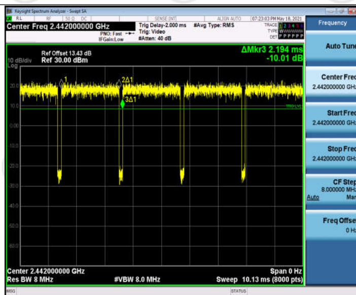
11G_Ant1_2442
