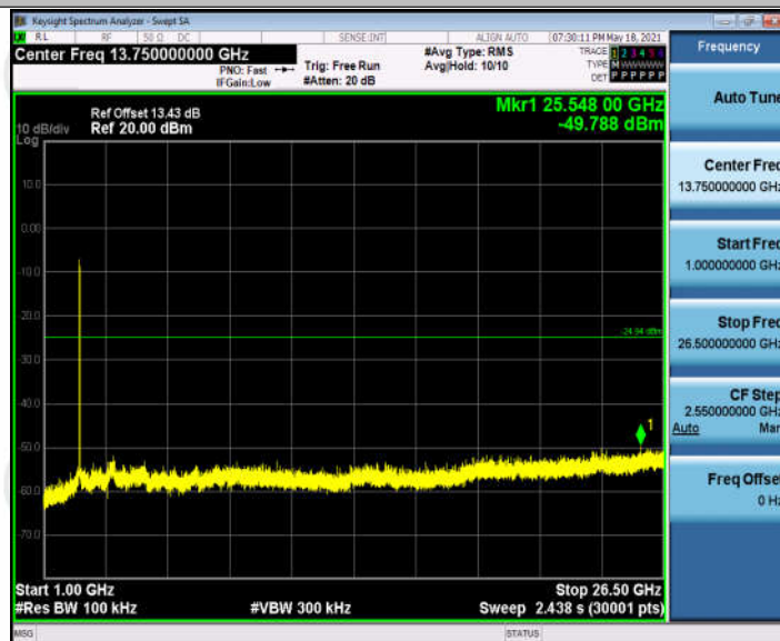
11G_Ant1_2472_1000~26500
