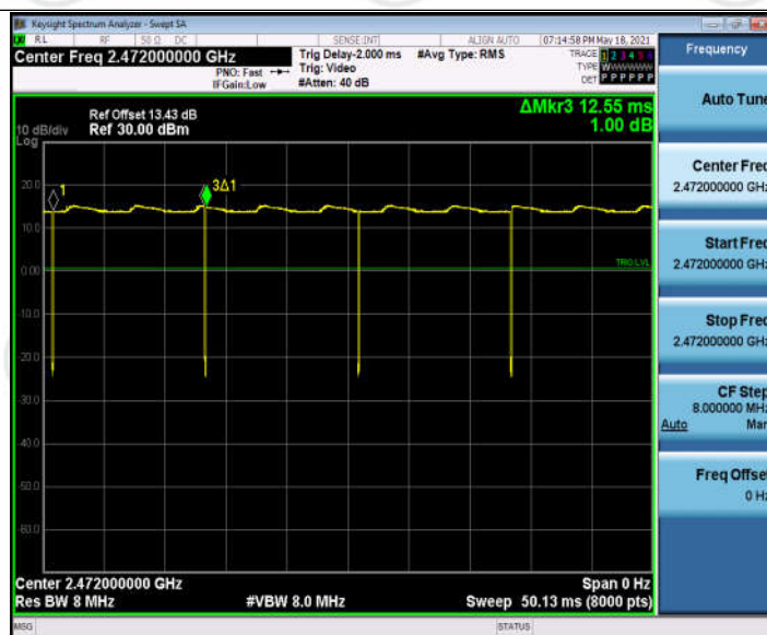
11B_Ant1_2472
