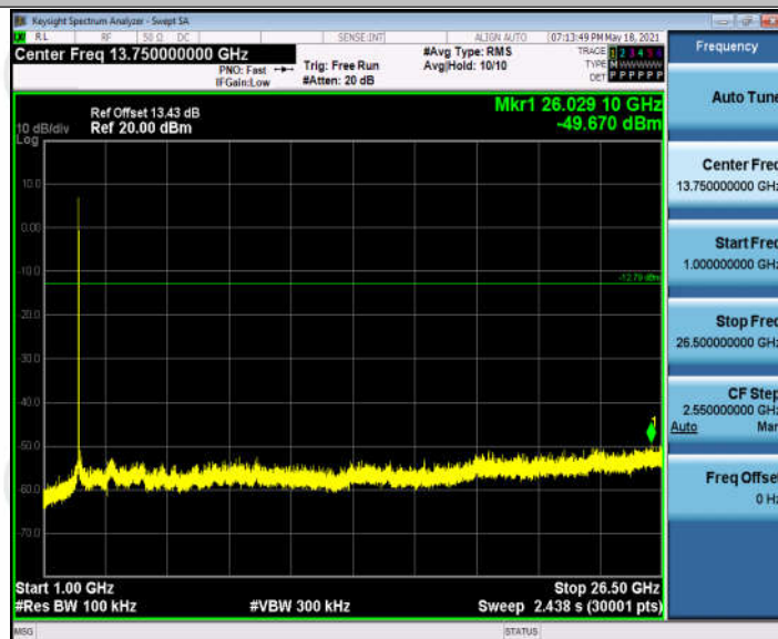
11B_Ant1_2442_1000~26500
