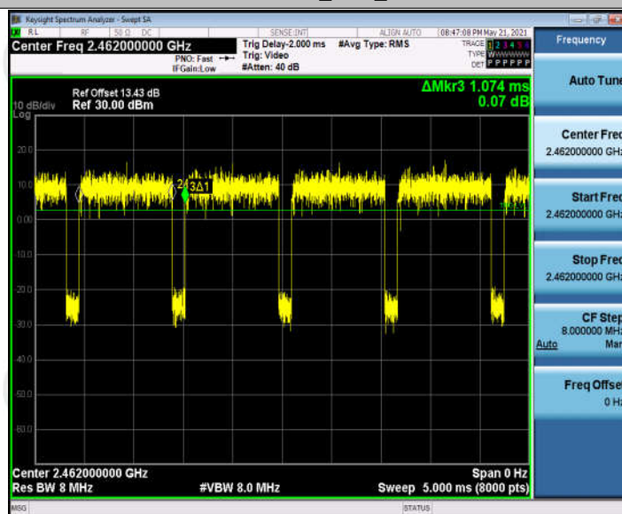
11N40SISO_Ant1_2462
