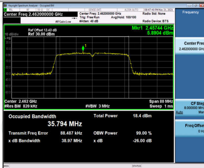
11N40SISO_Ant1_2462
