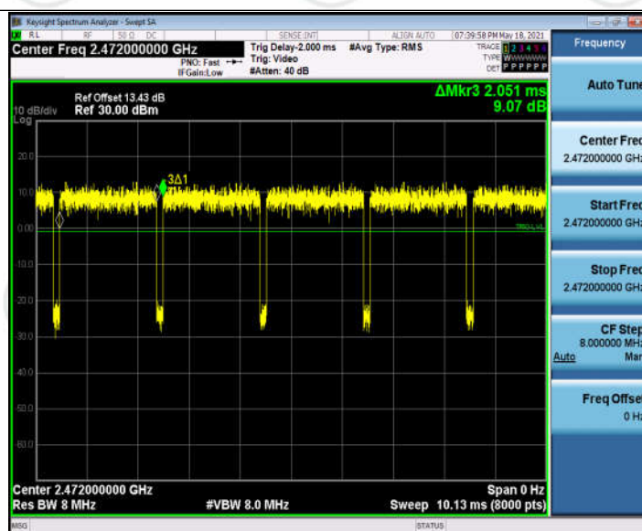
11N20SISO_Ant1_2472
