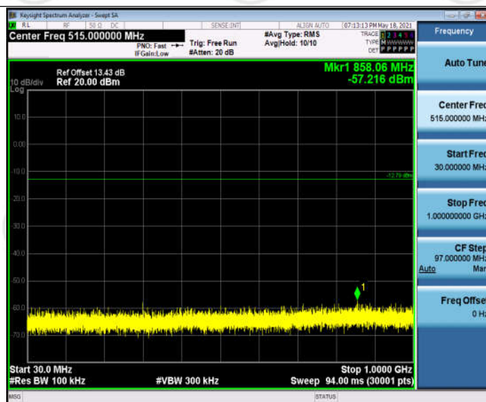
11B_Ant1_2442_30~1000
