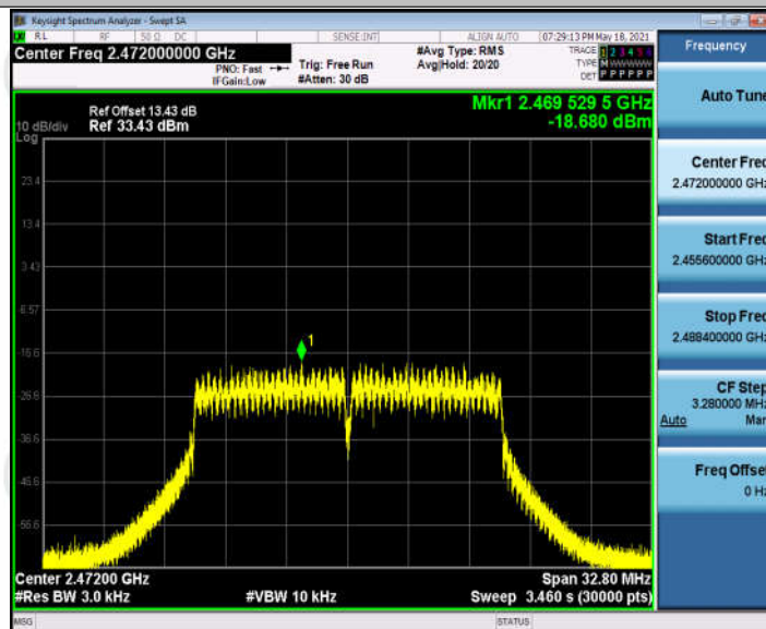
11G_Ant1_2472
