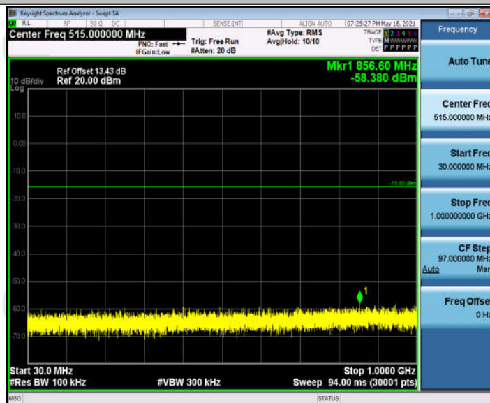
11G_Ant1_2442_30~1000
