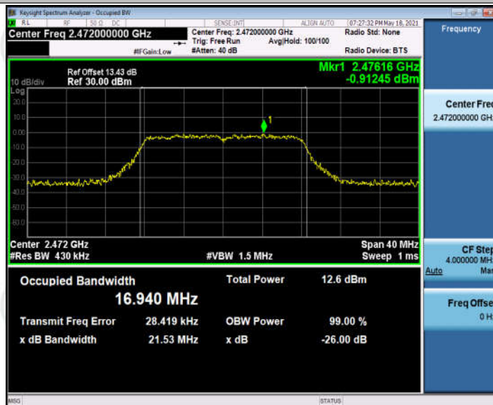
11G_Ant1_2472
