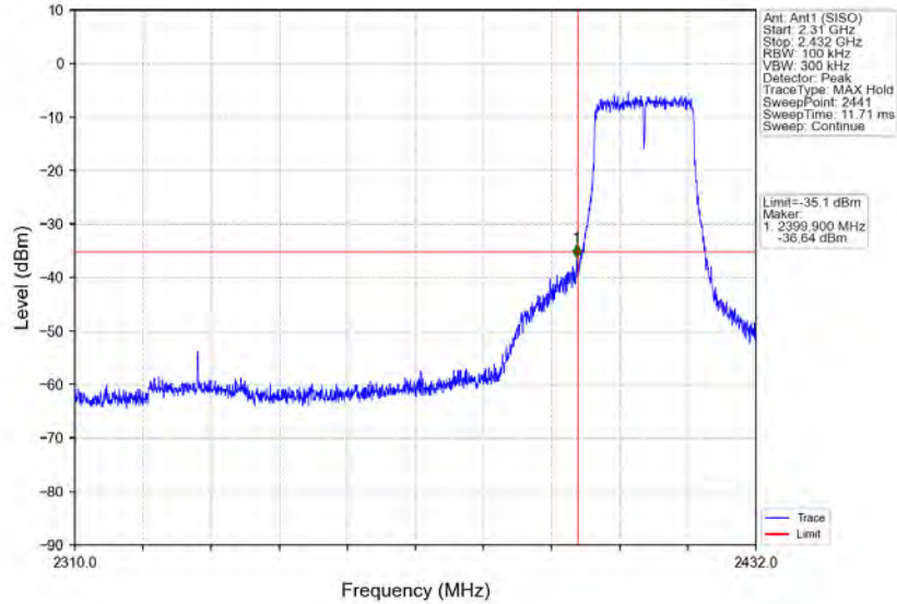
802.11n(HT20)_LCH_2412MHz_Ant1 (SISO)_NTNV
