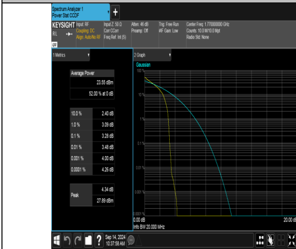
Band66-20MHz-QPSK-132572-1RB#0-PASS
