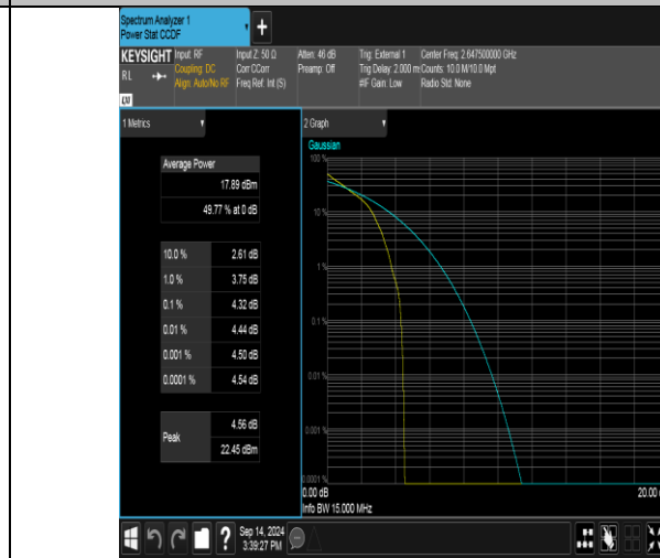
Band41(2535-2655)-15MHz-QPSK-41165-1RB#0-PASS
