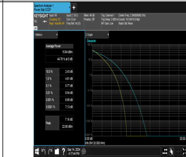
Band41(2535-2655)-20MHz-QPSK-40590-100RB#0-PASS
