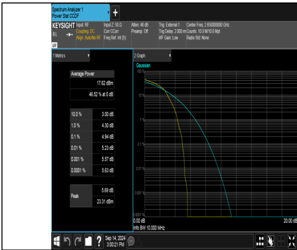
Band41(2535-2655)-10MHz-16QAM-41190-1RB#0-PASS
