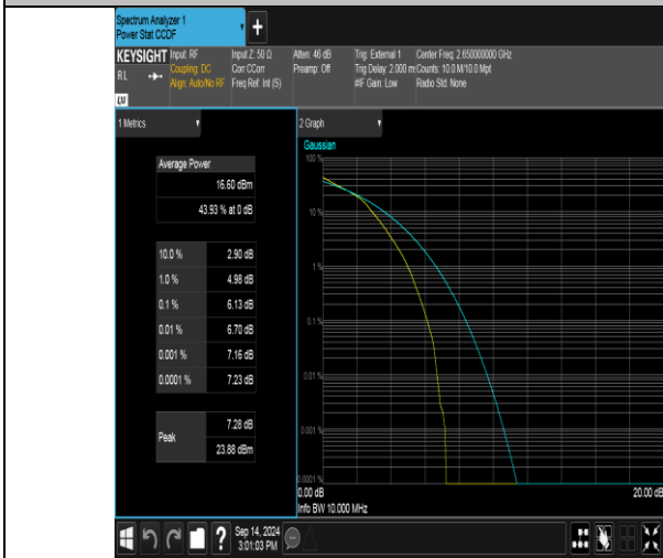
Band41(2535-2655)-10MHz-16QAM-41190-50RB#0-PASS
