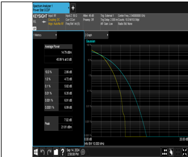
Band41(2535-2655)-10MHz-16QAM-40090-50RB#0-PASS
