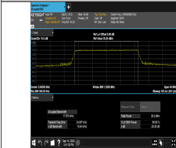
Band41(2535-2655)-20MHz-QPSK-41140-100RB#0-PASS
