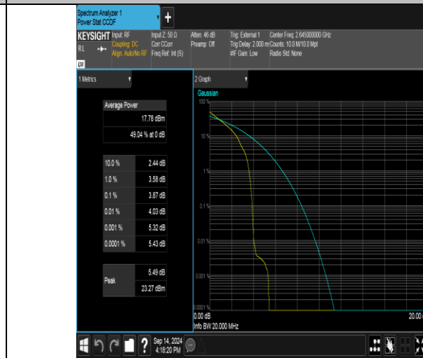
Band41(2535-2655)-20MHz-QPSK-41140-1RB#0-PASS
