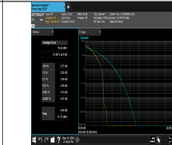
Band41(2535-2655)-20MHz-QPSK-40140-1RB#0-PASS
