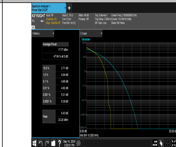
Band41(2535-2655)-10MHz-QPSK-41190-1RB#0-PASS
