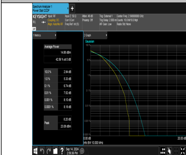
Band41(2535-2655)-10MHz-16QAM-40590-50RB#0-PASS
