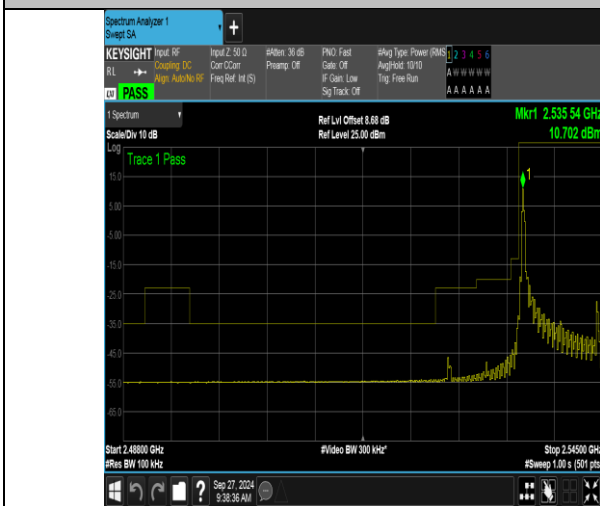
Band41_10MHz_QPSK_40090_1RB#0
