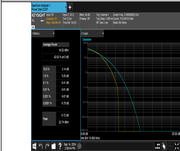
Band41(2535-2655)-10MHz-16QAM-40590-1RB#0-PASS
