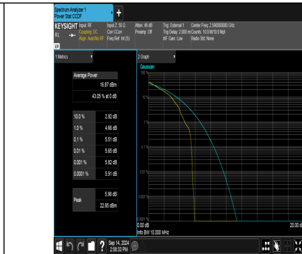
Band41(2535-2655)-10MHz-QPSK-40590-1RB#0-PASS
