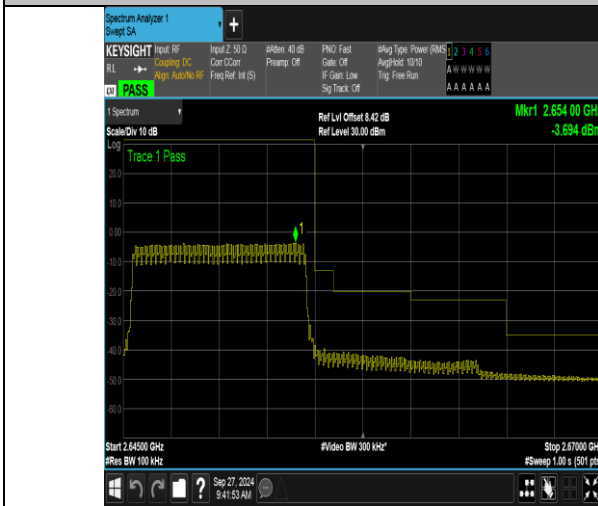
Band41_10MHz_QPSK_41190_50RB#0
