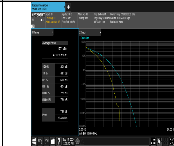
Band41(2535-2655)-10MHz-QPSK-40590-50RB#0-PASS
