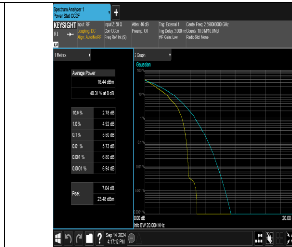
Band41(2535-2655)-20MHz-QPSK-40590-1RB#0-PASS
