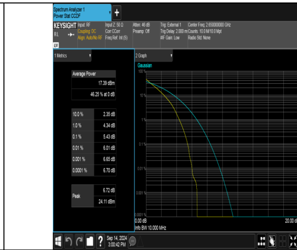
Band41(2535-2655)-10MHz-QPSK-41190-50RB#0-PASS
