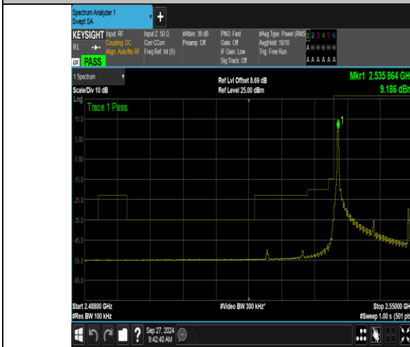
Band41_15MHz_QPSK_40115_1RB#0
