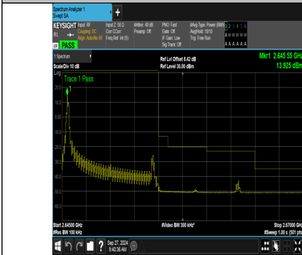
Band41_10MHz_QPSK_41190_1RB#0
