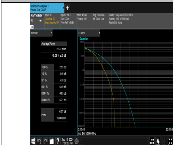
Band26(824-849)-3MHz-QPSK-26915-1RB#0-PASS
