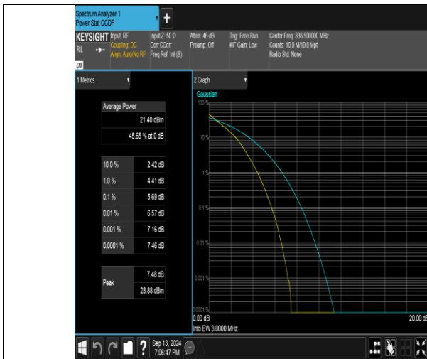
Band26(824-849)-3MHz-QPSK-26915-15RB#0-PASS
