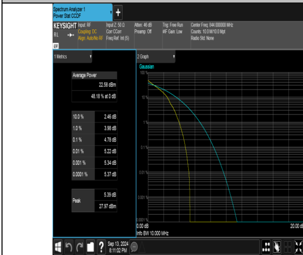
Band26(824-849)-10MHz-QPSK-26990-1RB#0-PASS
