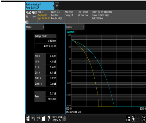
Band26(824-849)-10MHz-QPSK-26840-50RB#0-PASS
