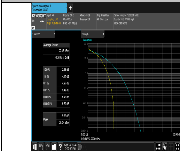
Band26(824-849)-3MHz-QPSK-27025-1RB#0-PASS
