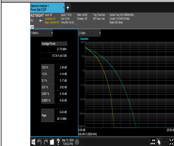
Band26(824-849)-3MHz-QPSK-26805-15RB#0-PASS
