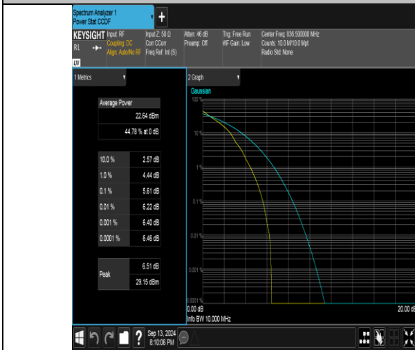
Band26(824-849)-10MHz-QPSK-26915-1RB#0-PASS
