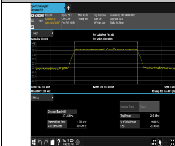
Band26(824-849)-3MHz-QPSK-27025-15RB#0-PASS
