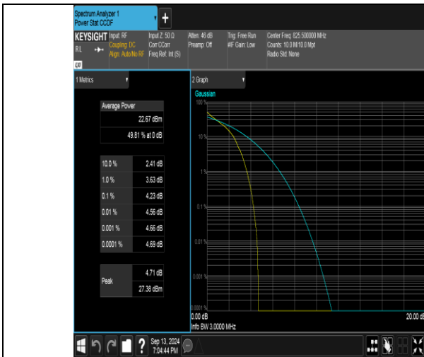
Band26(824-849)-3MHz-QPSK-26805-1RB#0-PASS
