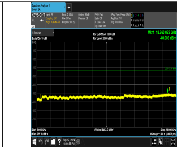
Band4_20MHz_16QAM_2050_1RB#99_3000-20000_3000-20000
