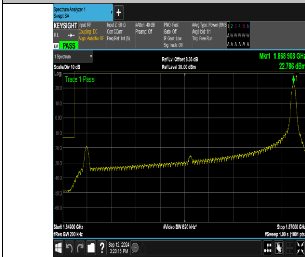
Band2_20MHz_QPSK_18700_1RB#99
