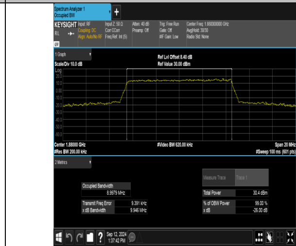
Band2-10MHz-16QAM-18900-50RB#0-PASS
