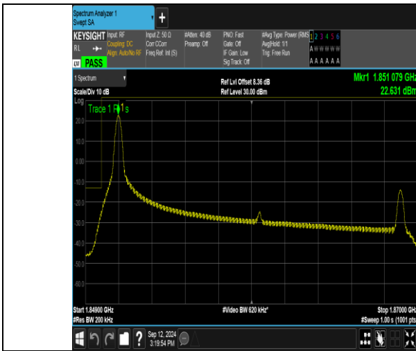
Band2_20MHz_QPSK_18700_1RB#0
