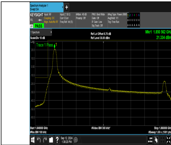
Band2_10MHz_QPSK_18650_1RB#0
