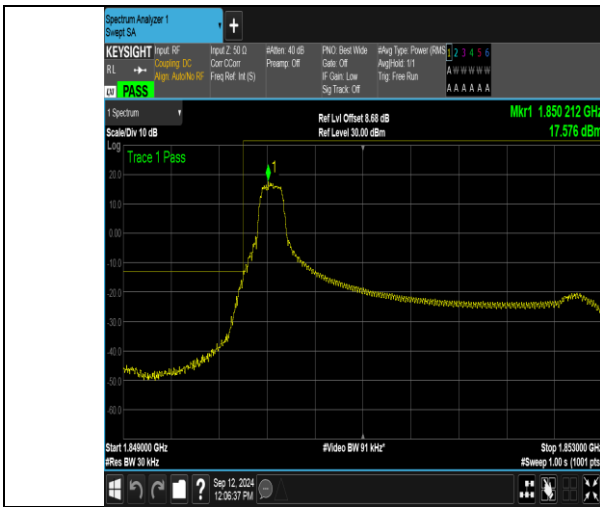
Band2_3MHz_QPSK_18615_1RB#0
