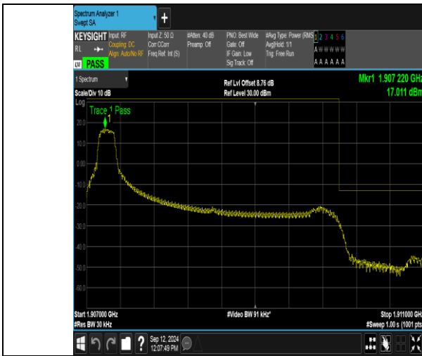
Band2_3MHz_QPSK_19185_1RB#0
