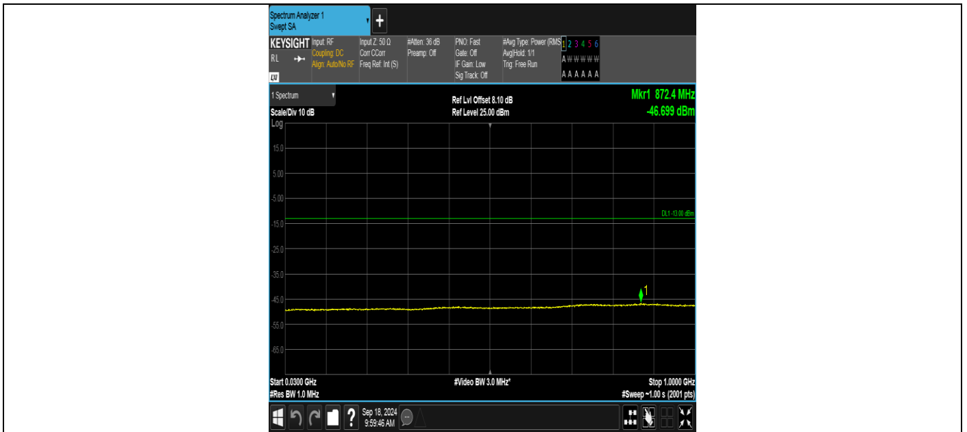
Band2-9400-1-30~1000MHz-PASS
