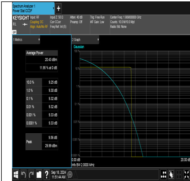
GSM1900-810-0-PASS
