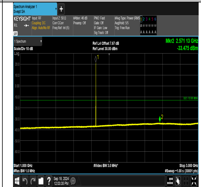
GSM1900-512-0-1000~3000MHz-PASS
