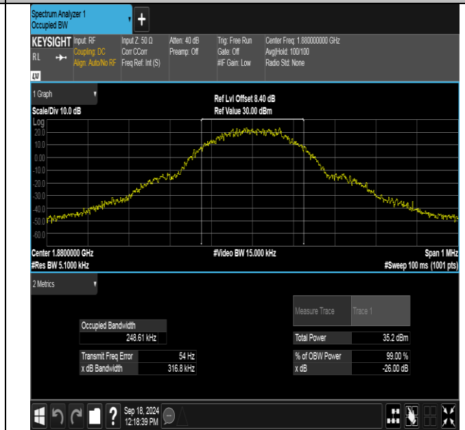
GPRS1900-661-0-PASS
