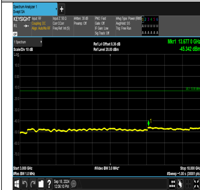
GSM1900-810-0-3000~18000MHz-PASS
