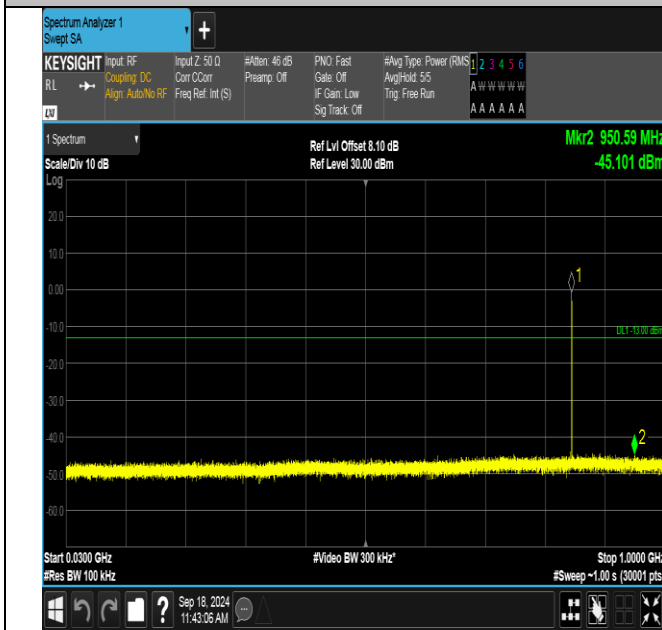
GPRS850-251-5-30~1000MHz-PASS
