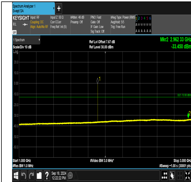
GPRS1900-810-0-1000~3000MHz-PASS
