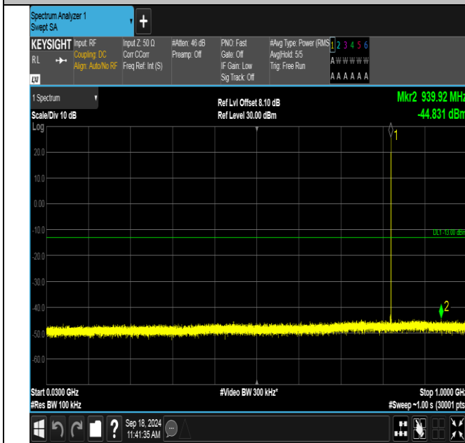
GPRS850-128-5-30~1000MHz-PASS
