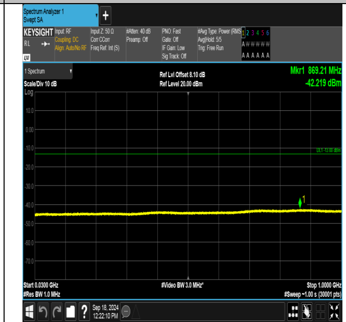
GPRS1900-810-0-30~1000MHz-PASS
