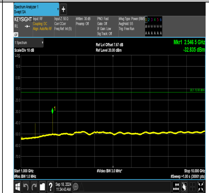
GSM850-251-5-1000~10000MHz-PASS
