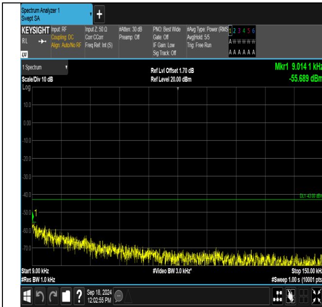
GSM1900-512-0-0.009~0.15MHz-PASS
