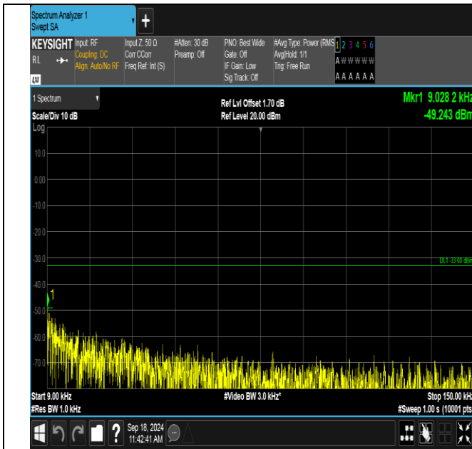
GPRS850-251-5-0.009~0.15MHz-PASS
