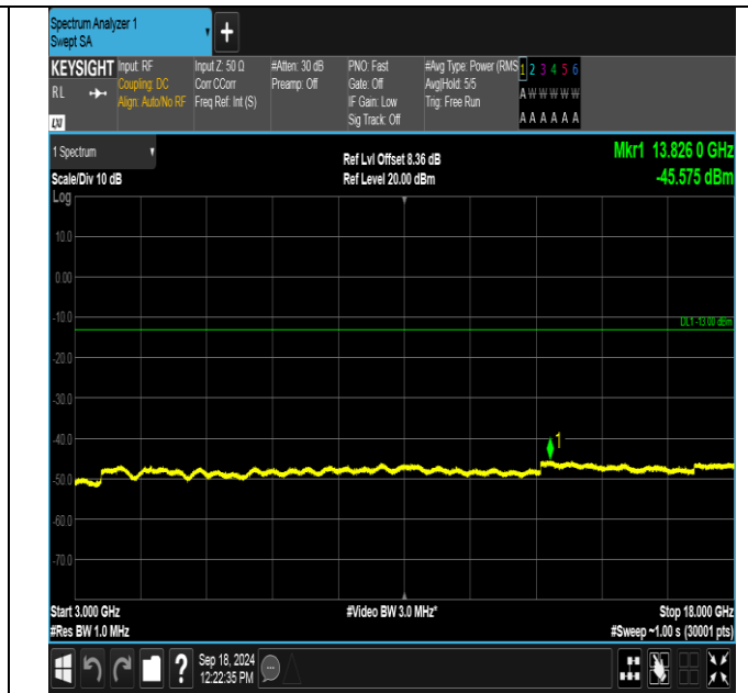
GPRS1900-810-0-3000~18000MHz-PASS
