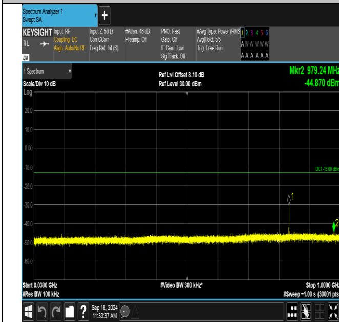
GSM850-190-5-30~1000MHz-PASS
