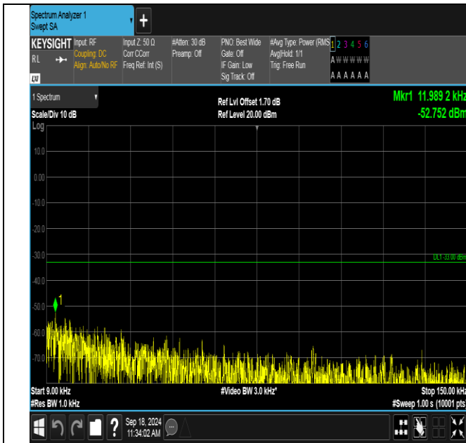
GSM850-251-5-0.009~0.15MHz-PASS
