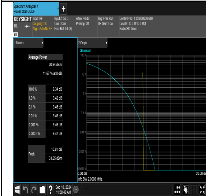
GSM1900-512-0-PASS
