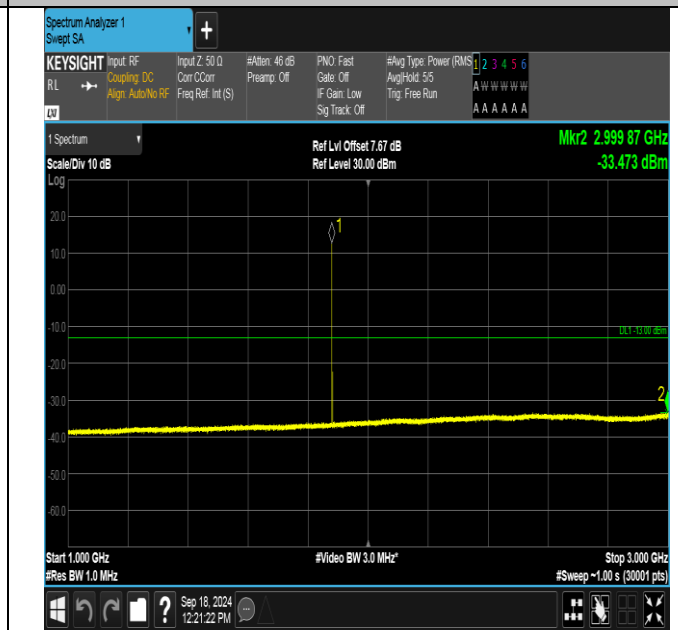
GPRS1900-661-0-1000~3000MHz-PASS
