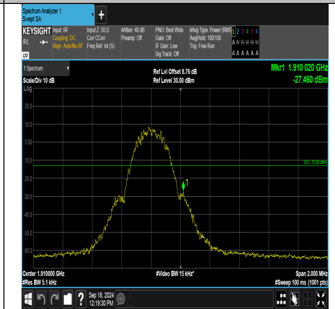
GPRS1900-810-0-PASS
