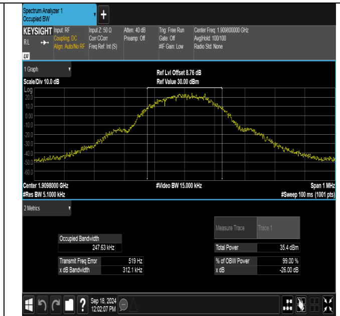
GSM1900-810-0-PASS
