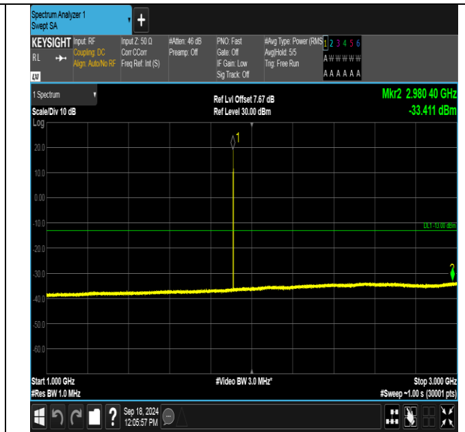
GSM1900-810-0-1000~3000MHz-PASS
