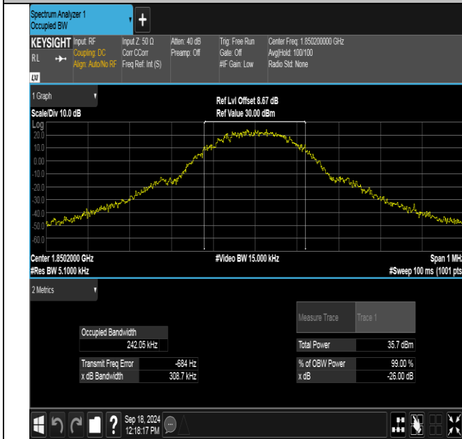
GPRS1900-512-0-PASS
