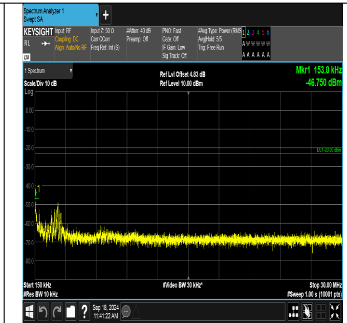
GPRS850-128-5-0.15~30MHz-PASS
