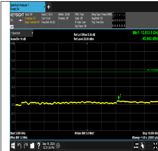
GPRS1900-661-0-3000~18000MHz-PASS
