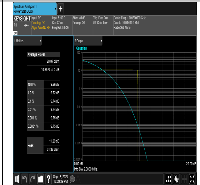
GPRS1900-810-0-PASS
