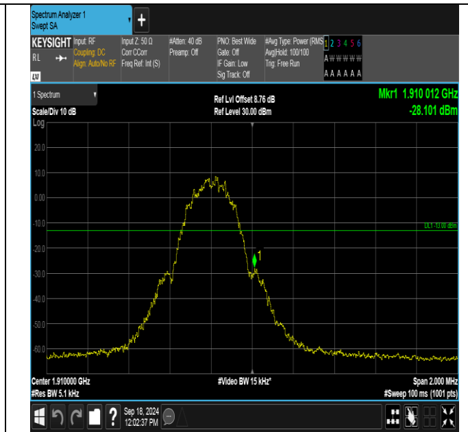
GSM1900-810-0-PASS
