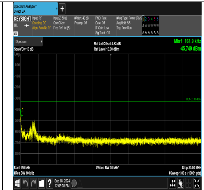
GSM1900-512-0-0.15~30MHz-PASS
