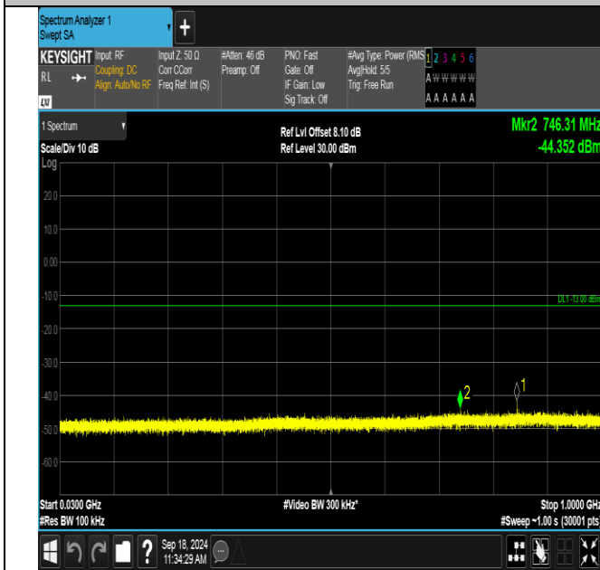
GSM850-251-5-30~1000MHz-PASS
