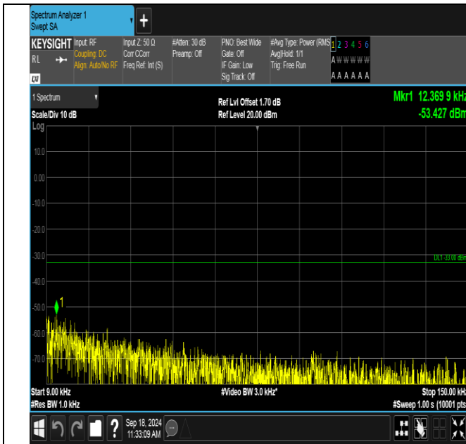
GSM850-190-5-0.009~0.15MHz-PASS
