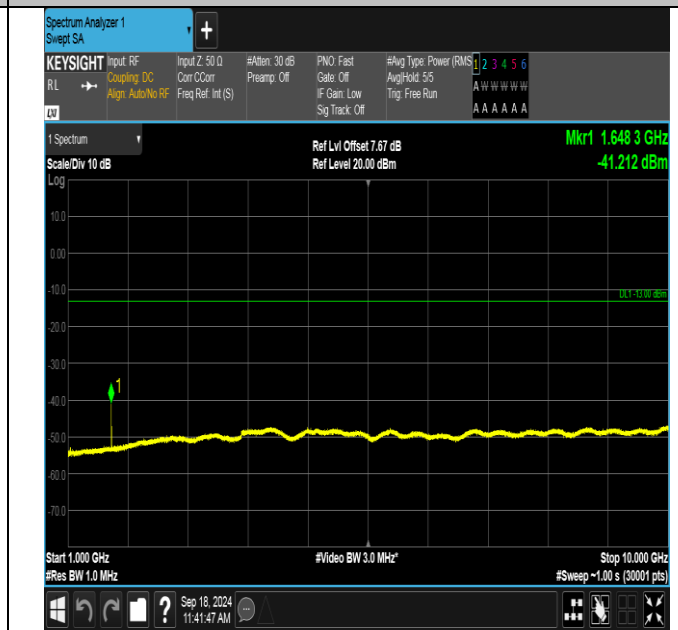
GPRS850-128-5-1000~10000MHz-PASS
