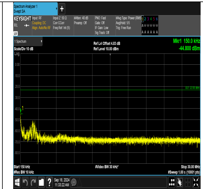
GSM850-190-5-0.15~30MHz-PASS
