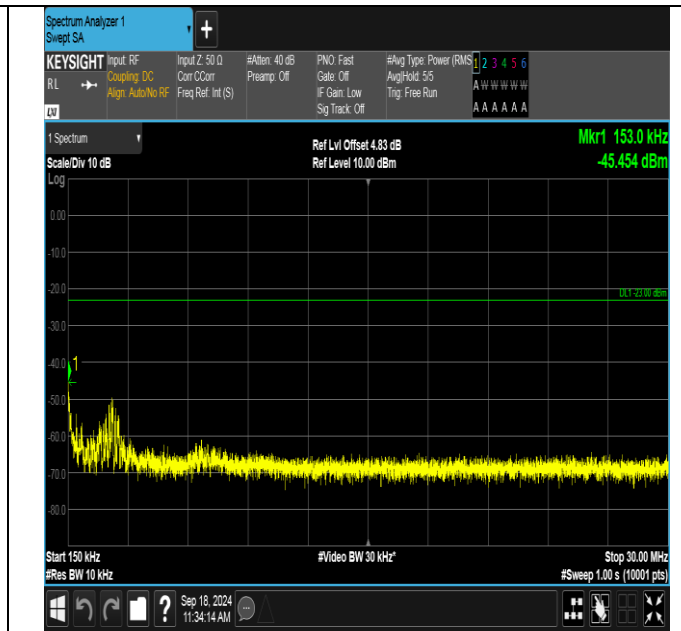
GSM850-251-5-0.15~30MHz-PASS
