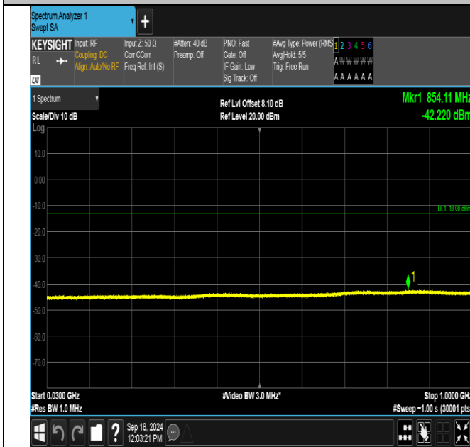
GSM1900-512-0-30~1000MHz-PASS
