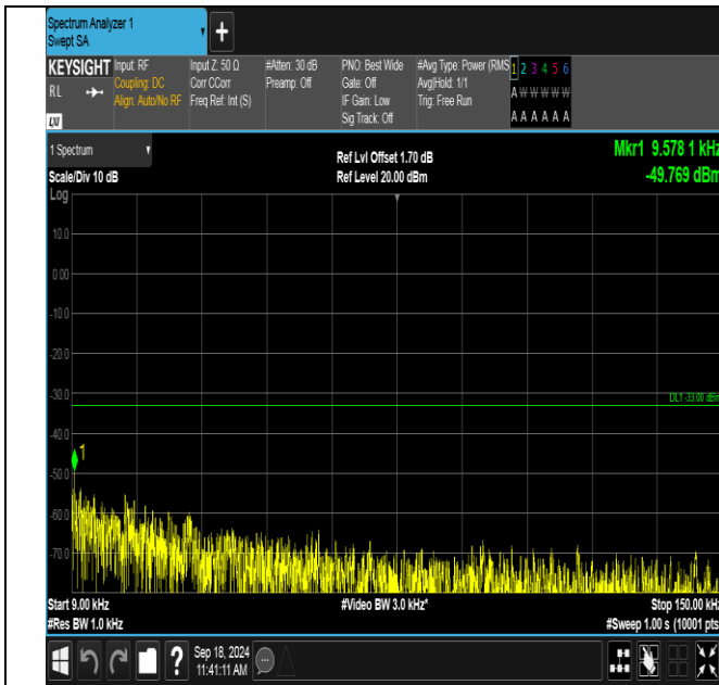
GPRS850-128-5-0.009~0.15MHz-PASS
