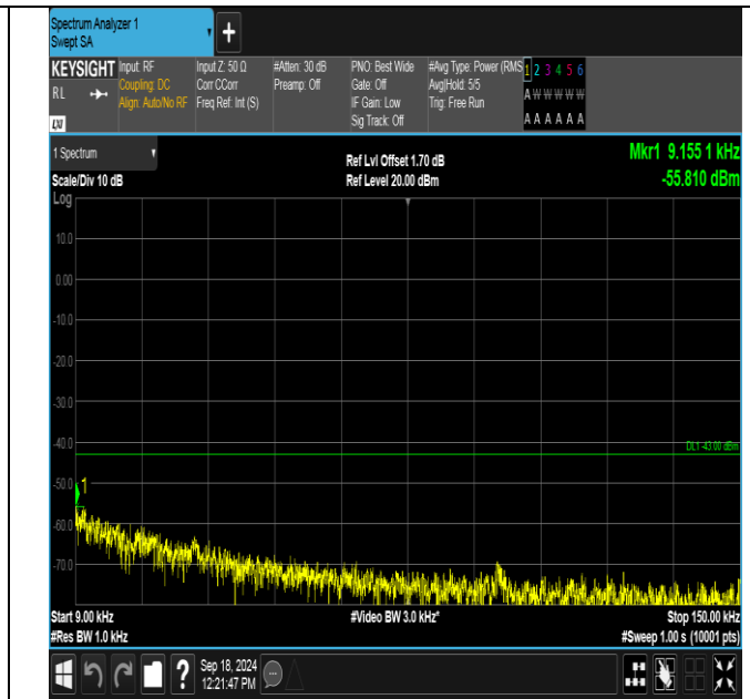
GPRS1900-810-0-0.009~0.15MHz-PASS
