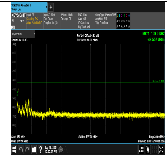
GPRS1900-661-0-0.15~30MHz-PASS
