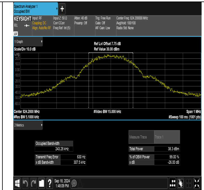
GPRS850-128-5-PASS
