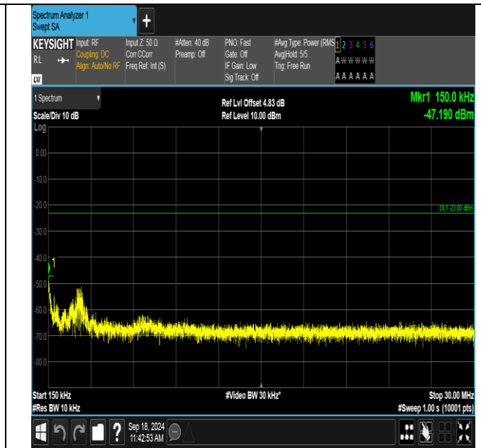
GPRS850-251-5-0.15~30MHz-PASS
