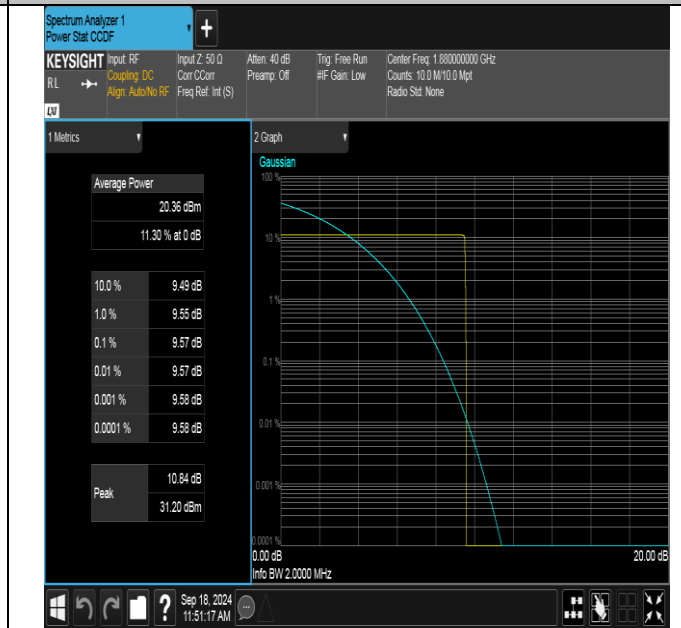
GSM1900-661-0-PASS
