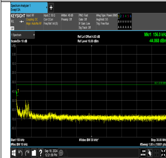
GPRS1900-810-0-0.15~30MHz-PASS
