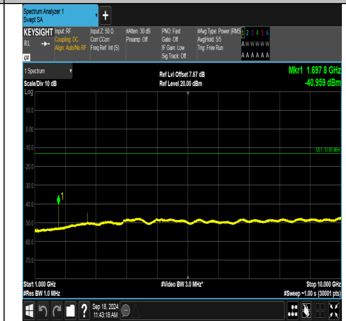
GPRS850-251-5-1000~10000MHz-PASS
