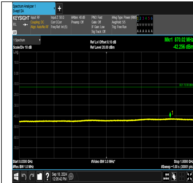
GSM1900-810-0-30~1000MHz-PASS
