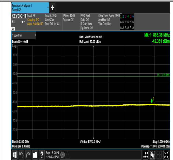
GSM1900-661-0-30~1000MHz-PASS
