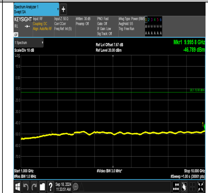
GSM850-190-5-1000~10000MHz-PASS
