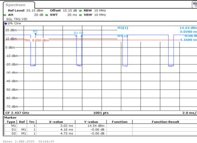
11G_Ant1_2437
