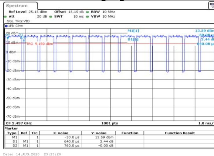
11N20_Ant1_2437
