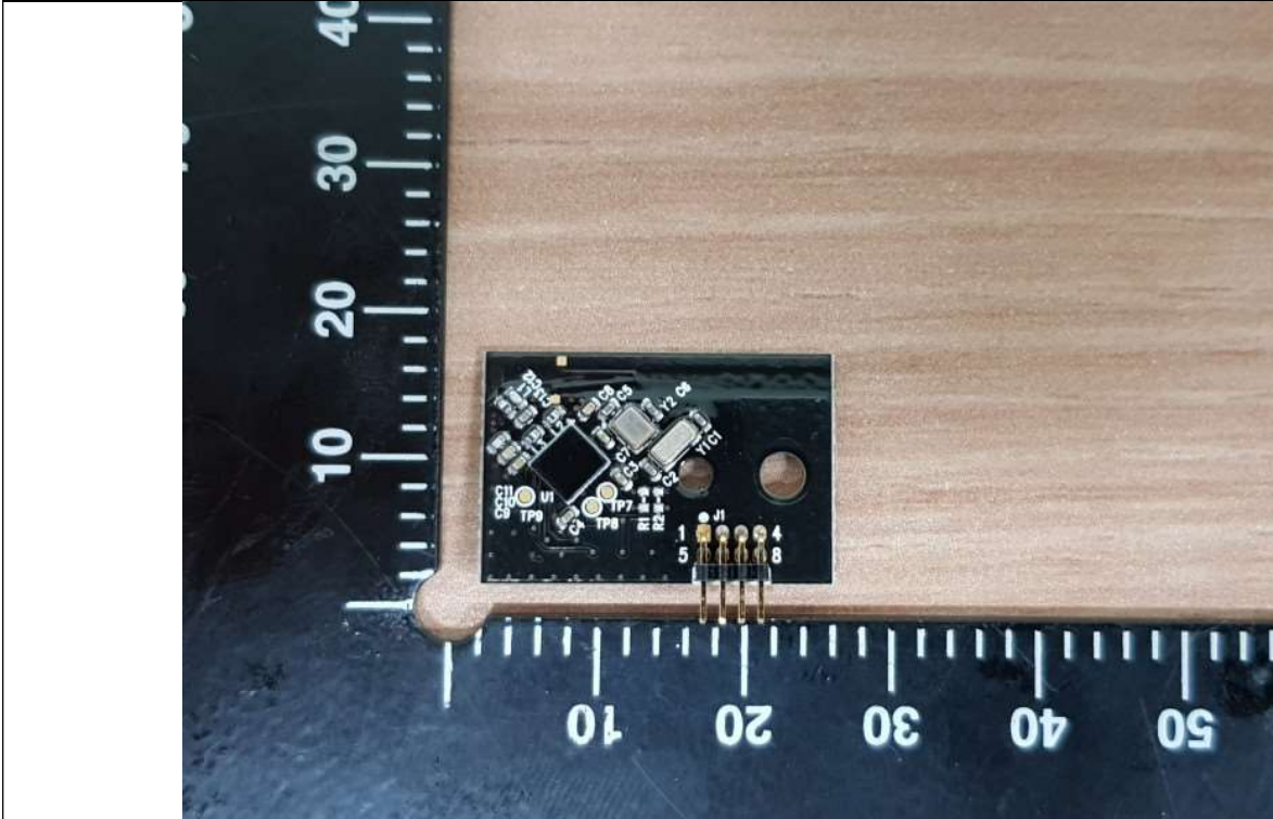
Bluetooth LE Module PCB - Rear
