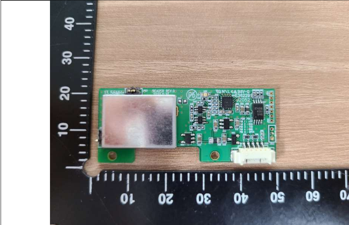
RFID Module PCB - Rear
