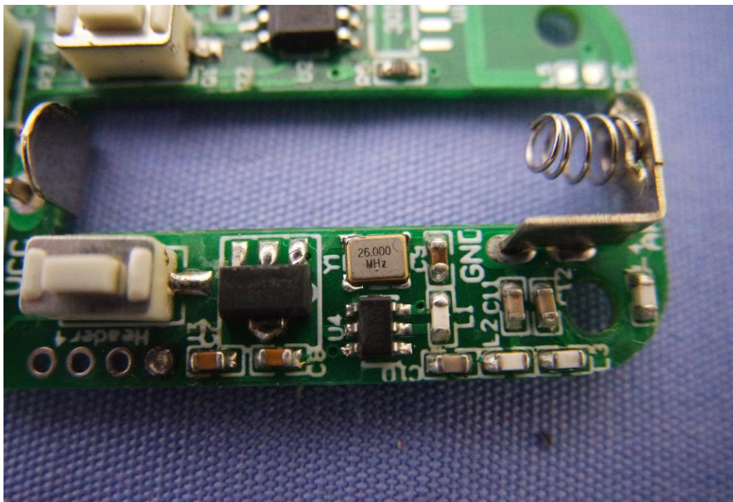
RF IC & Crystal
