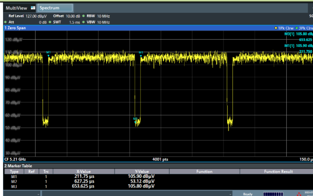
802.11ax-HE80
