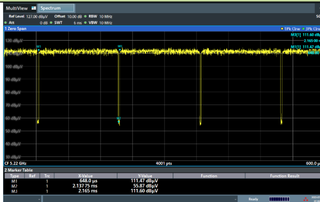
802.11ax-HE80
