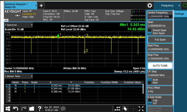
802.11ax-HE20
