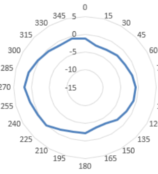
6525MHz-theta=90
