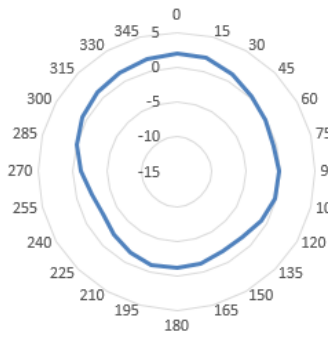
6125MHz-theta=90
