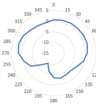
6525MHz-theta=90
