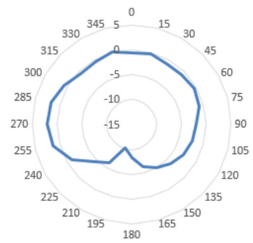
6925MHz-theta=90
