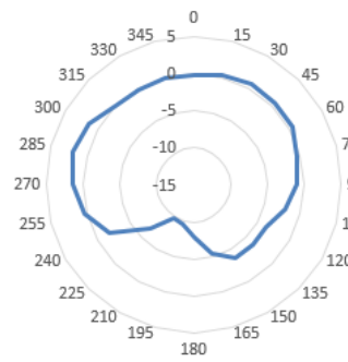
6125MHz-theta=90
