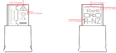
尺寸图
