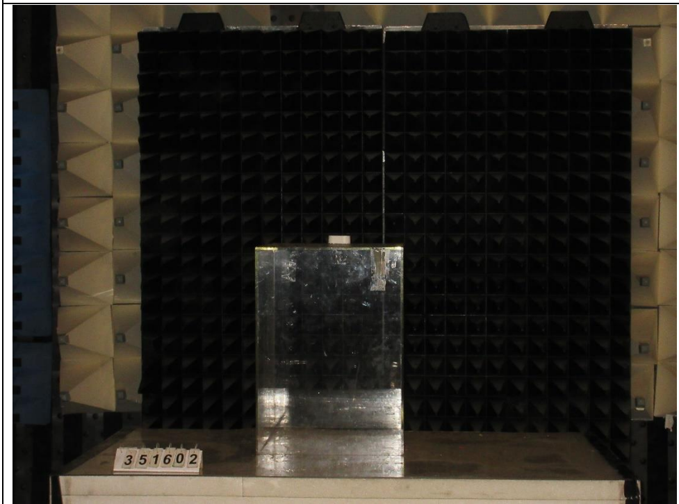
01. 禁用頻帶輻射發射之量測 1GHz 以下 (正面)
