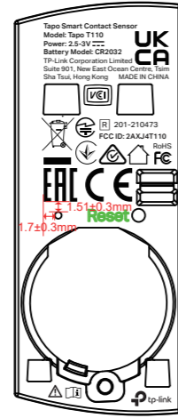
尺寸图
