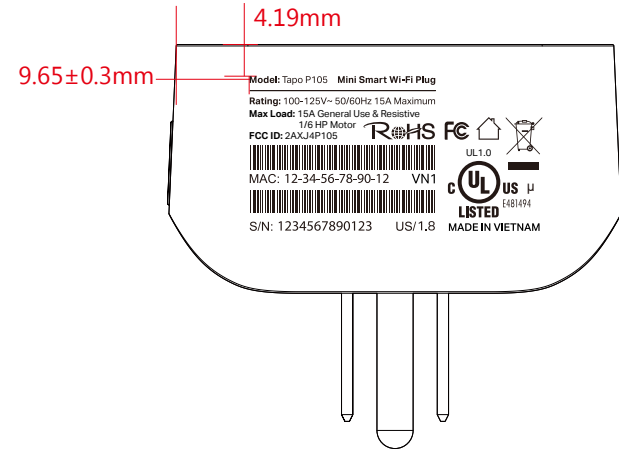
尺寸图
