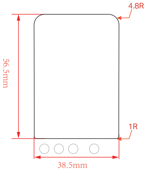
尺寸图
