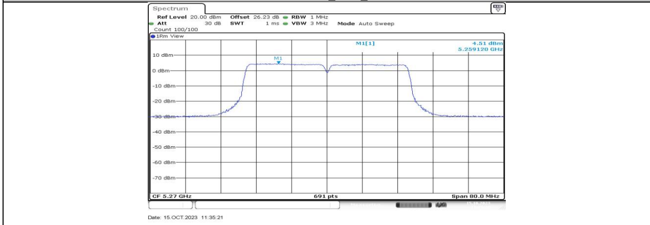
11N40MIMO_Ant4_5270
