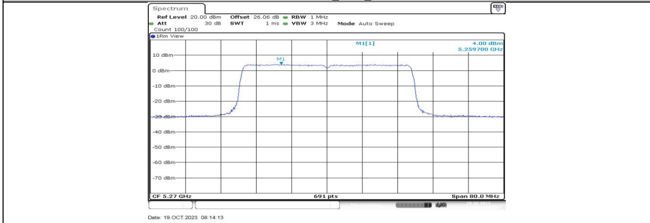
11AX40MIMO_Ant2_5270
