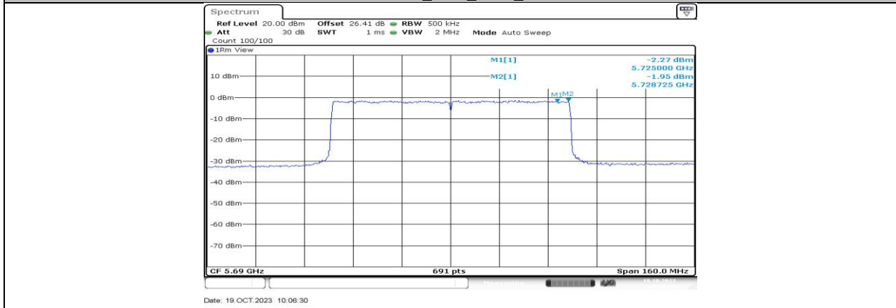
11AX80MIMO_Ant2_5690_UNII-3
