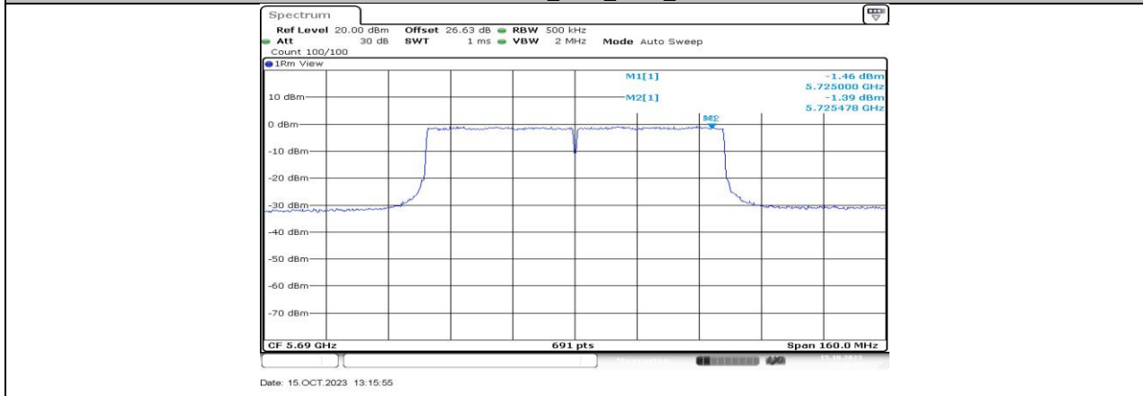
11AC80MIMO_Ant4_5690_UNII-3
